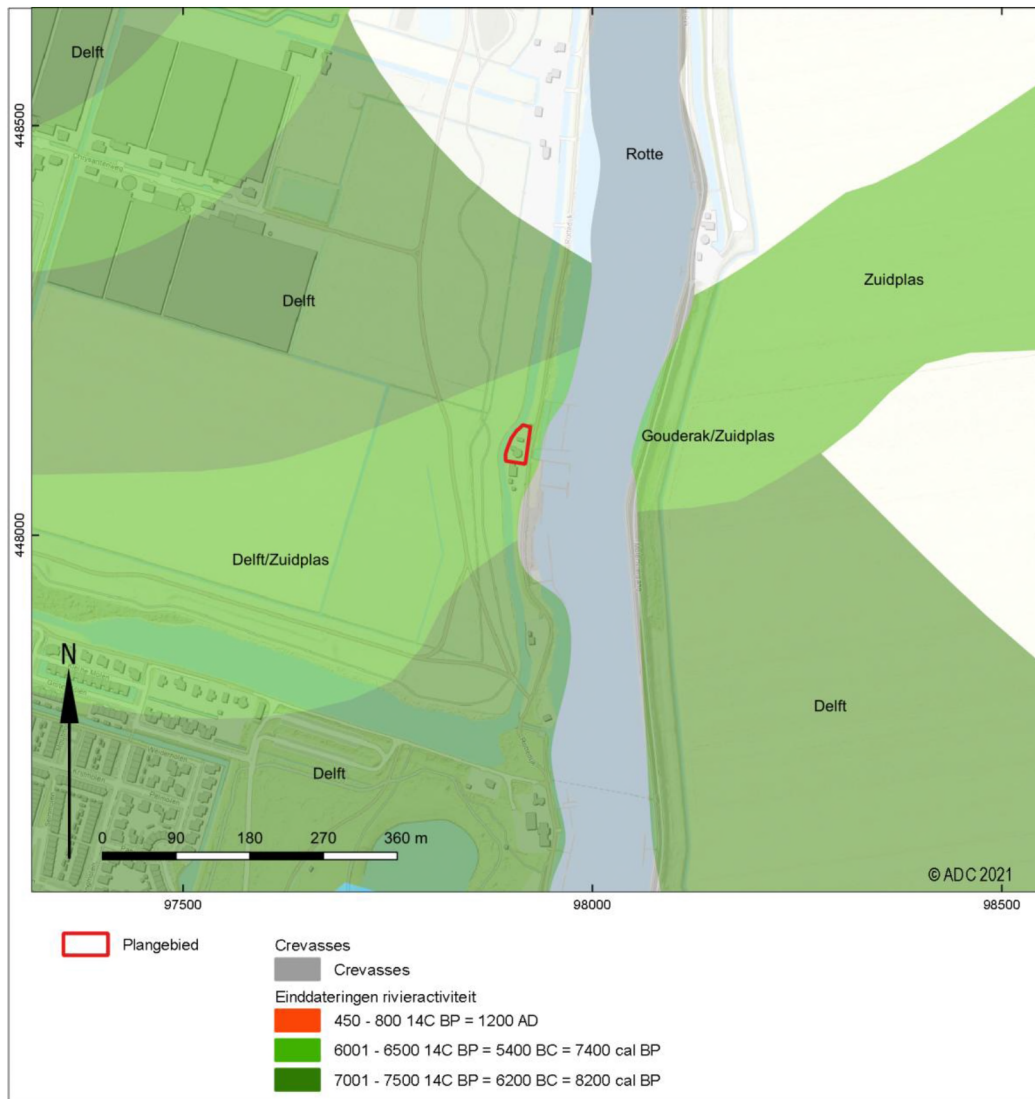
Afb. 5 Stroomgordelkaart
