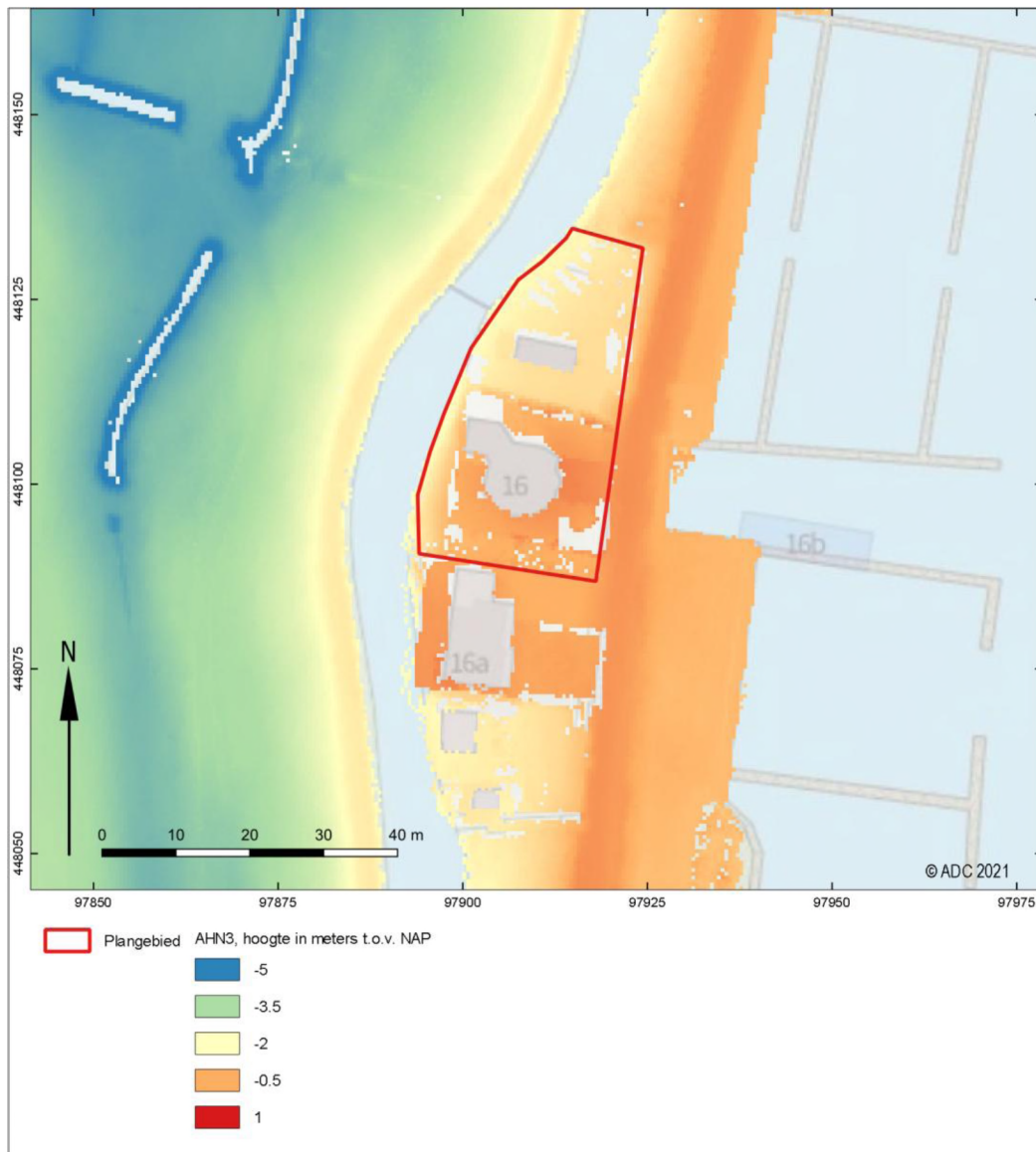
Afb. 7 AHN3 kaart
