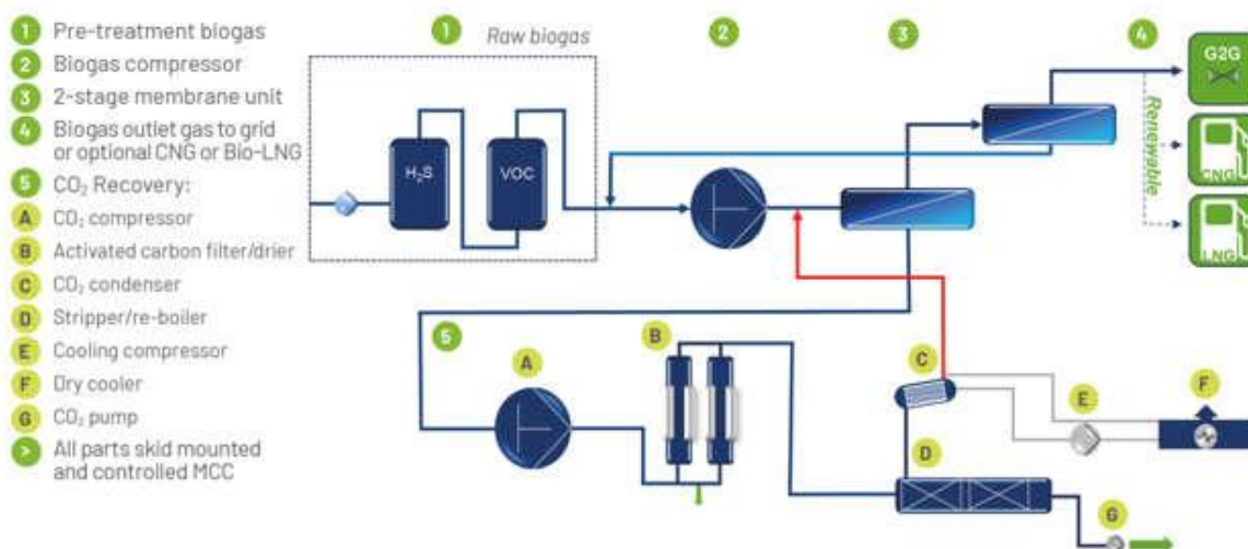
Figuur 5-2 Schematische weergave van gasopwerking met membranen
