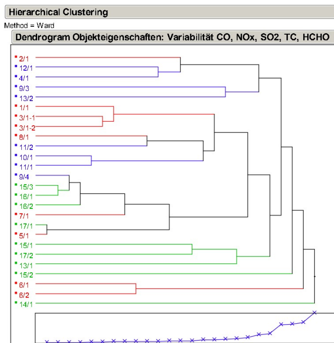
Abbildung 9: Dendrogramm Variabilität
