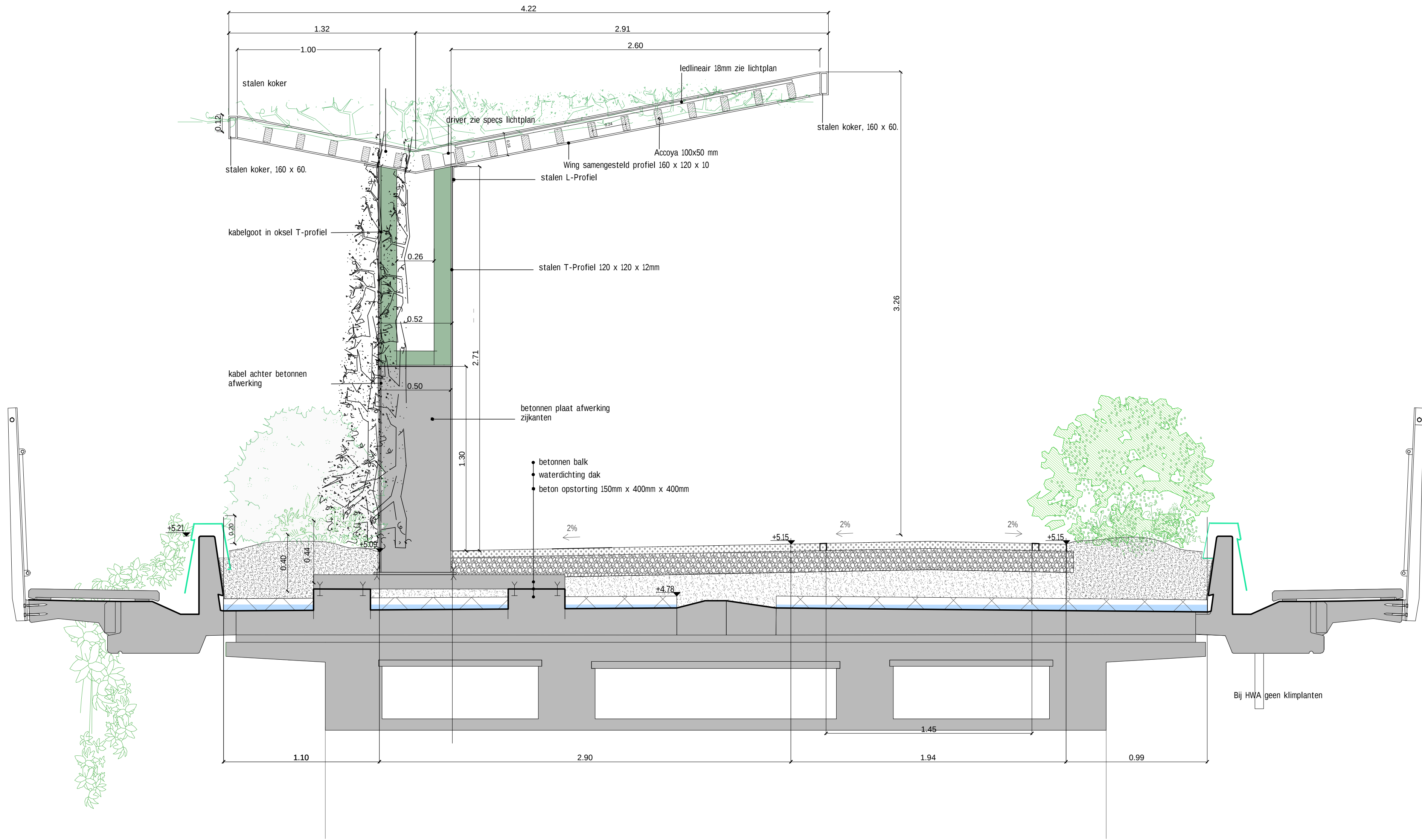
Doorsnede
