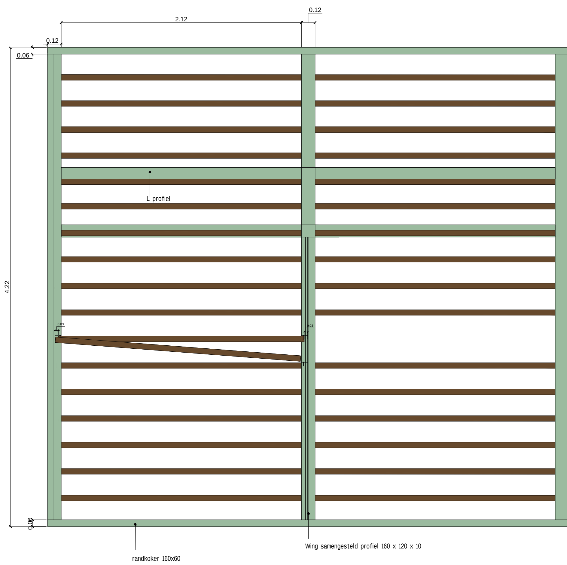
Bovenaanzicht
