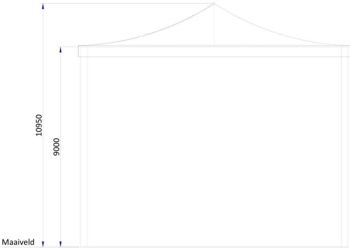
Voor aanzicht (1:100)
