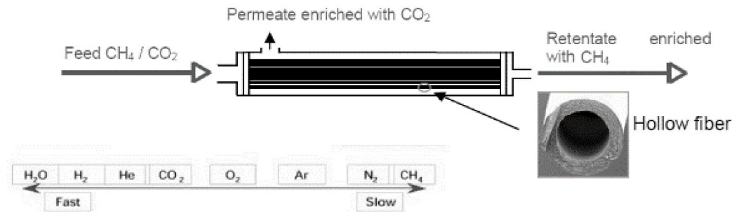
Figuur - Scheidingsprincipe membraantechnologie gebruikt in opwaardering van biogas
