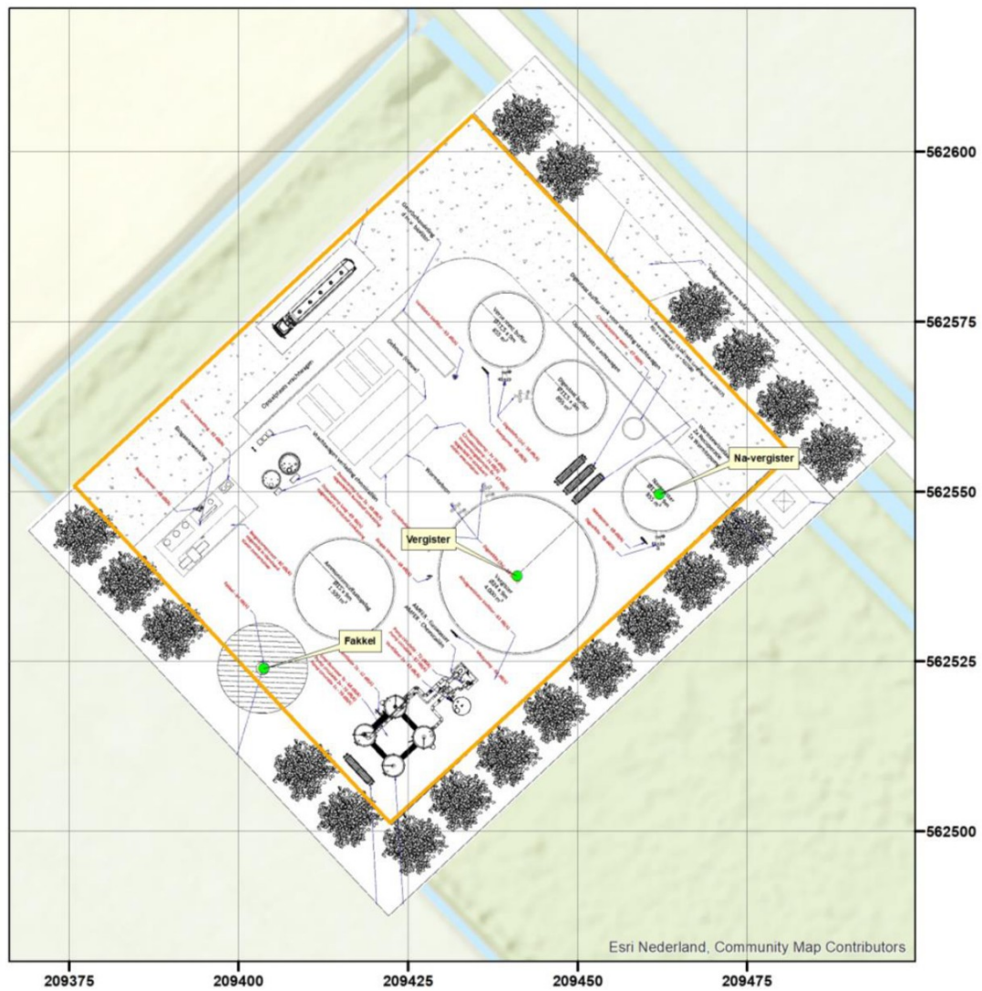
Figuur 1. Situatietekening
