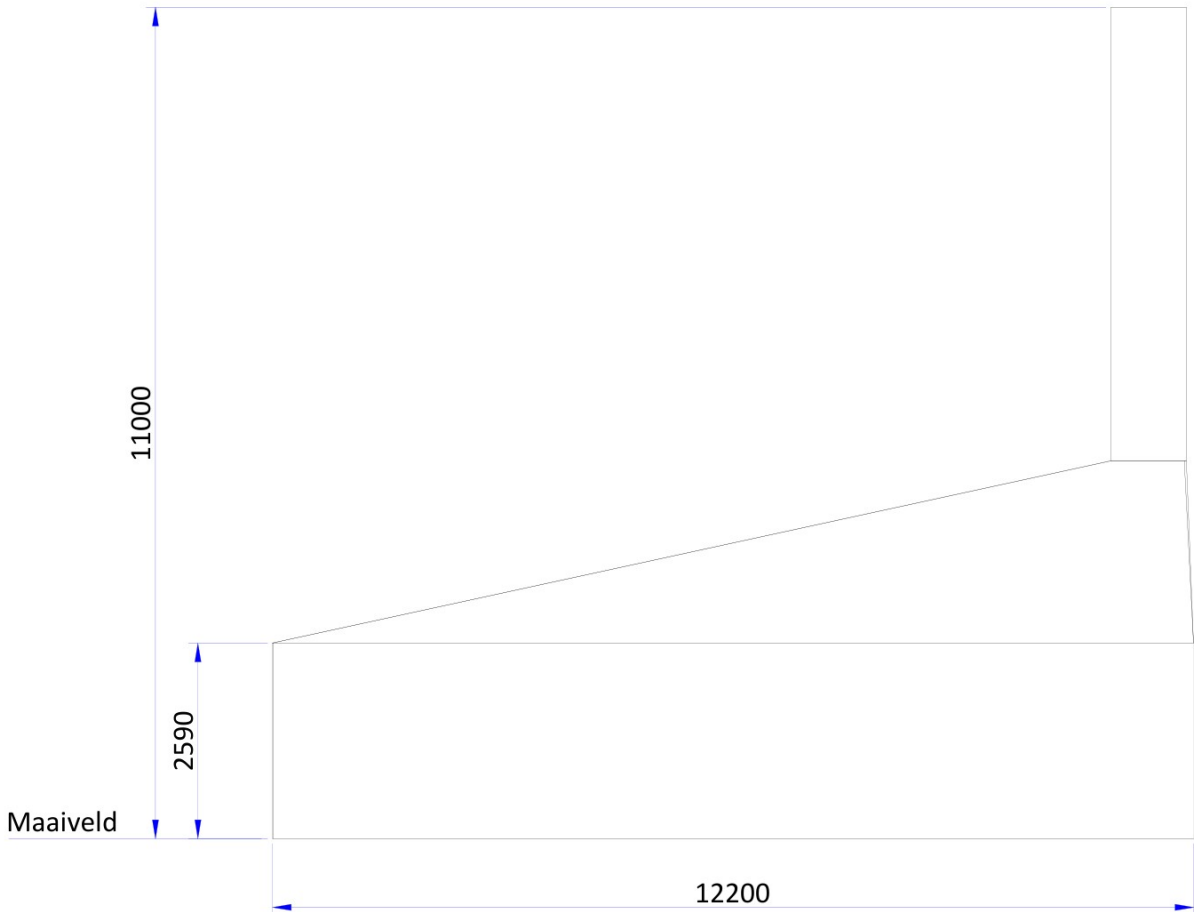
Voor aanzicht (1:100)
