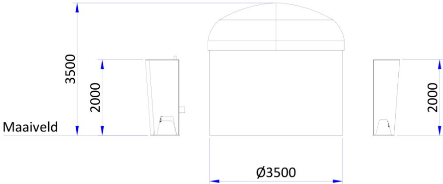
Voor aanzicht (1:100)
