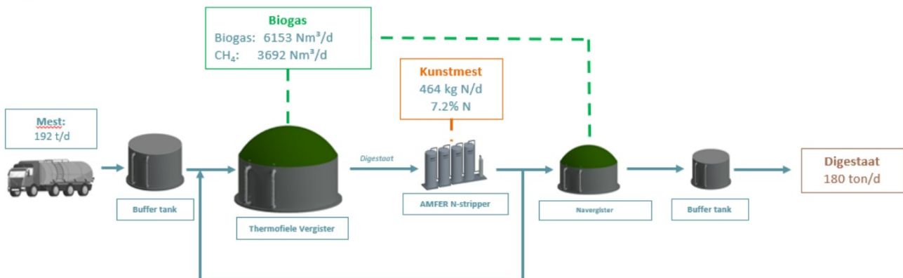
Figuur 4 – Processtroomschema
