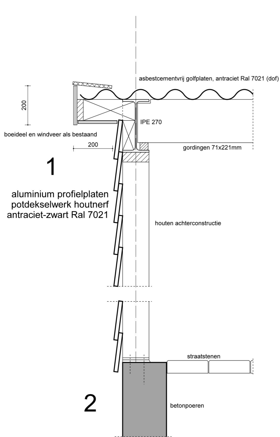
details kopgevel
