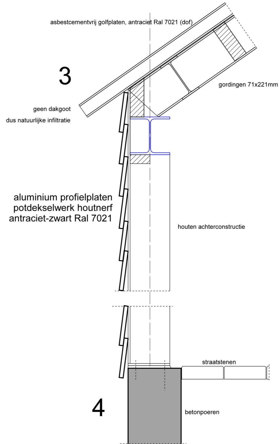
details langsgevel
