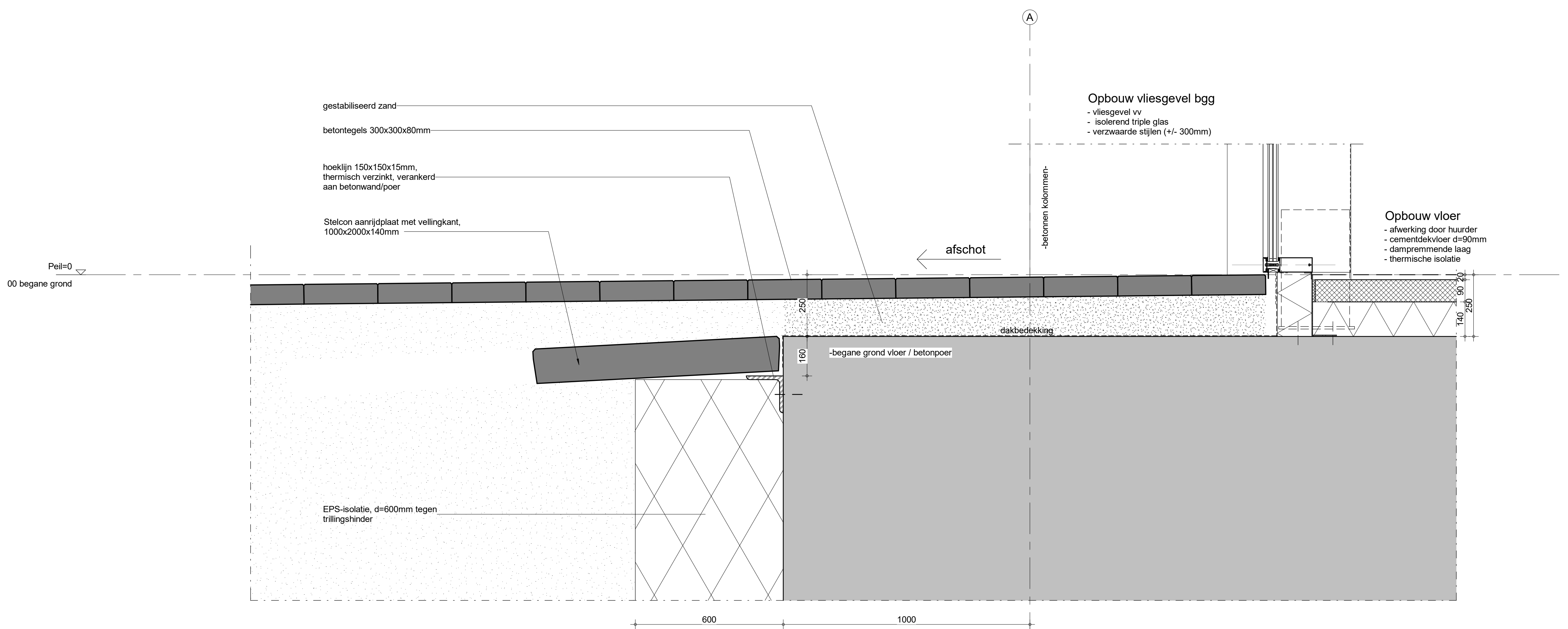
Fragment aanrijdplaten 1 : 50
