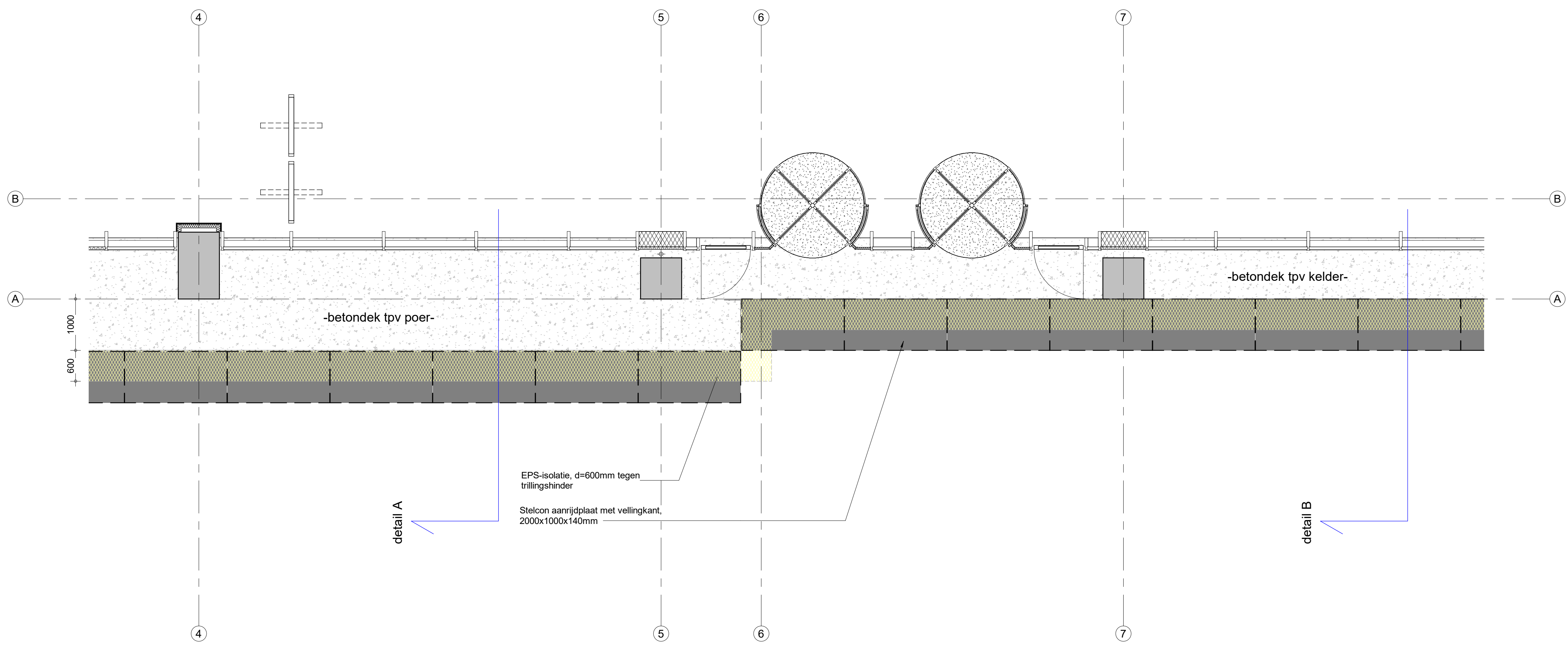
Fragment aanrijdplaten 1 : 50
