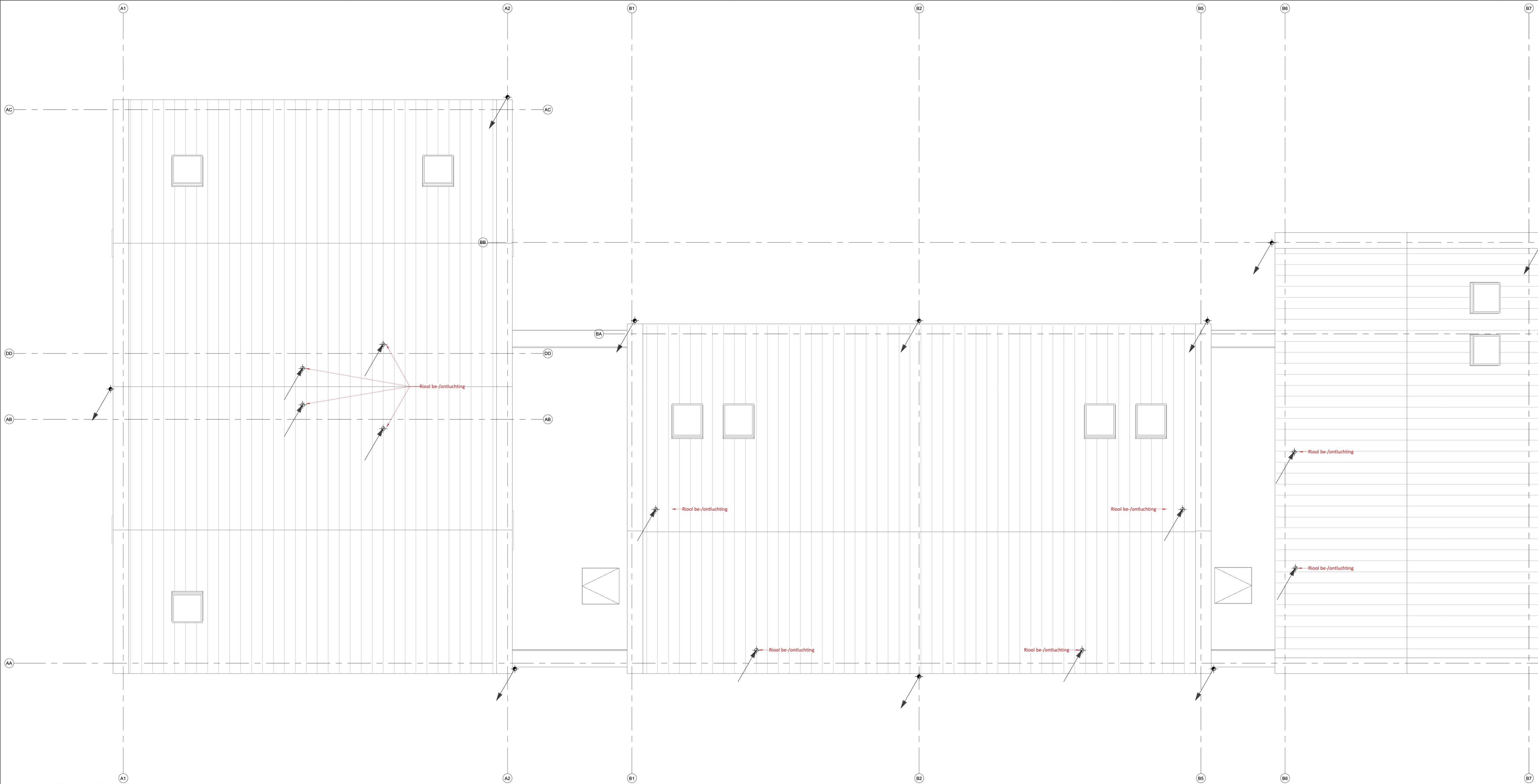
HWA & VWA dak 1 : 50
