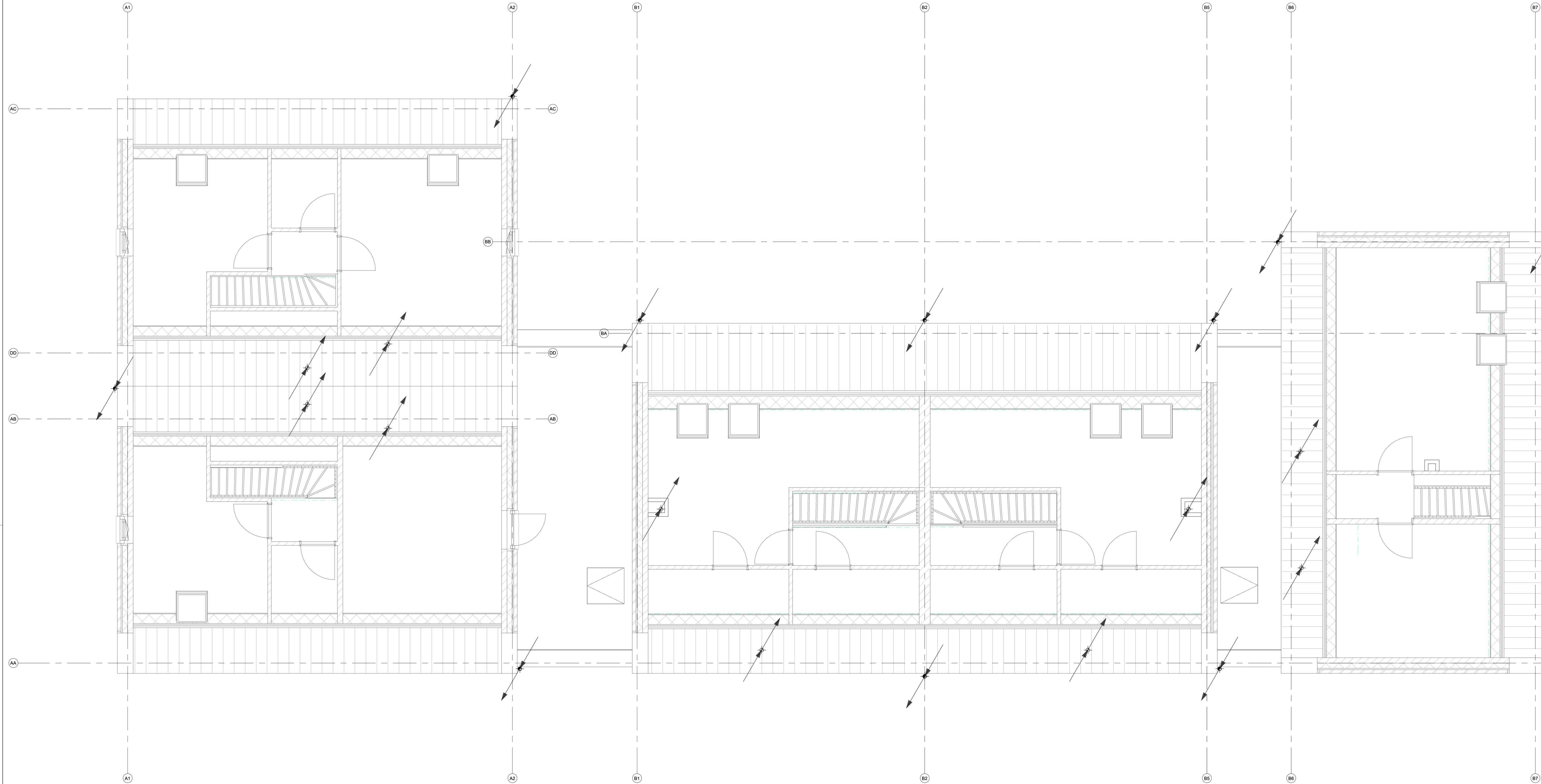
HWA & VWA 2e verdieping 1 : 50
