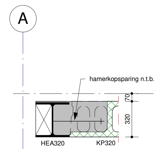
Detail -.01 Schaal: 1 : 20
