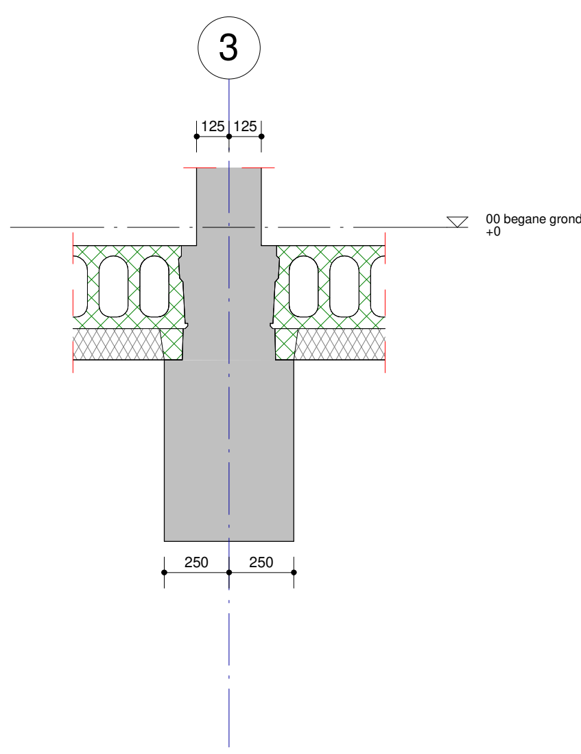
Detail 0.05 Schaal: 1 : 20
