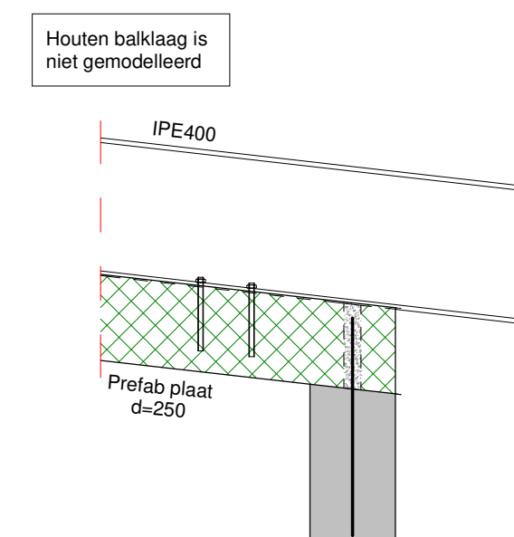
Detail 3.01 Schaal: 1 : 20
