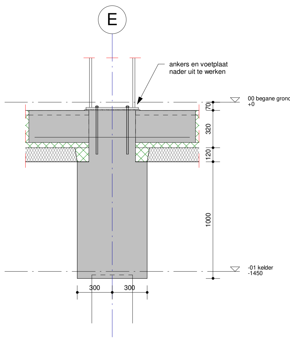
Detail 0.03 Schaal: 1 : 20
