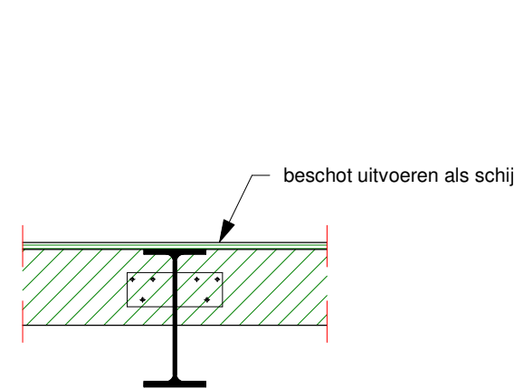
Detail 3.02 Schaal: 1 : 20
