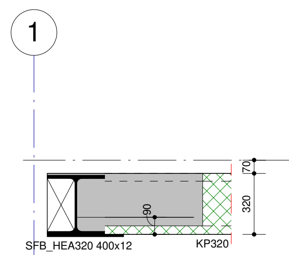
Detail -.02 Schaal: 1 : 20
