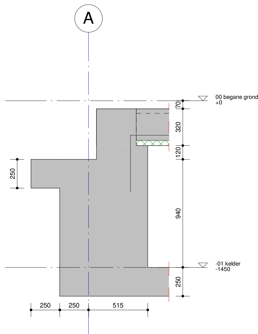
Detail 0.01 Schaal: 1 : 20
