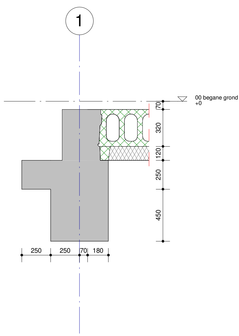
Detail 0.04 Schaal: 1 : 20
