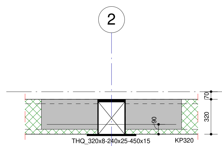
Detail -.03 Schaal: 1 : 20
