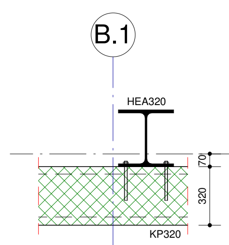
Detail -.05 Schaal: 1 : 20
