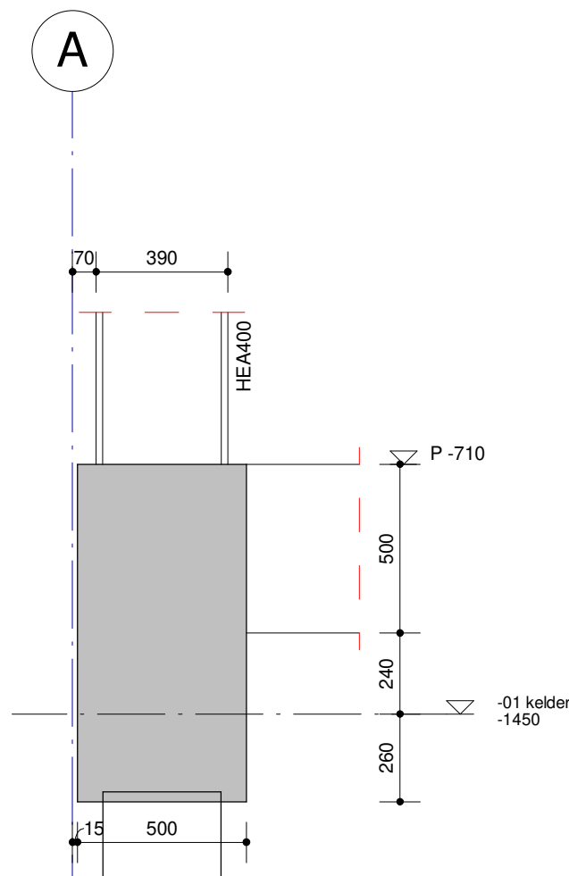
Detail 0.01 Schaal: 1 : 20
