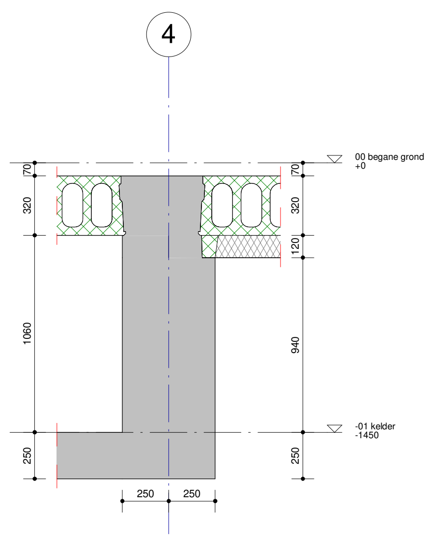
Detail 0.06 Schaal: 1 : 20
