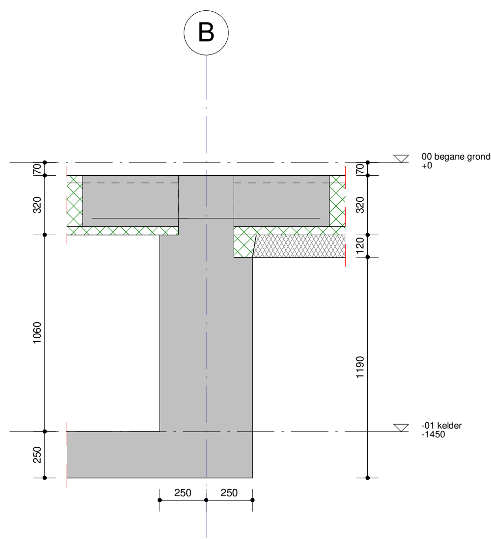
Detail 0.02 Schaal: 1 : 20
