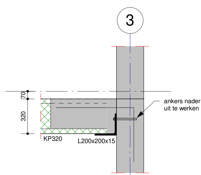
Detail -.04 Schaal: 1 : 20
