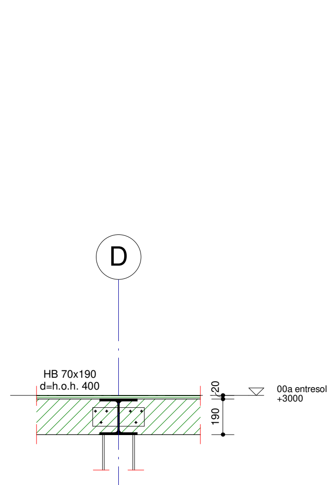
Detail 0.03 Schaal: 1 : 20
