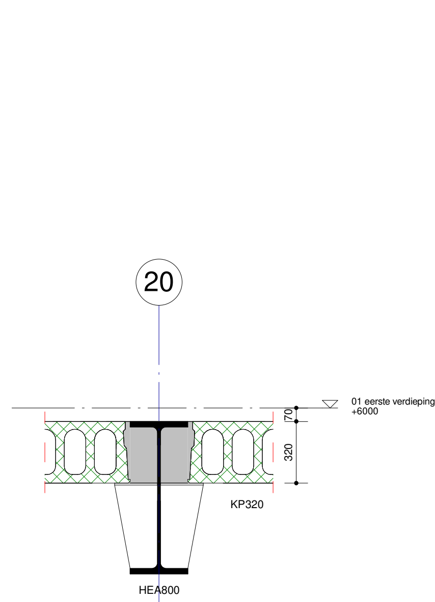
Detail 1.01 Schaal: 1 : 20
