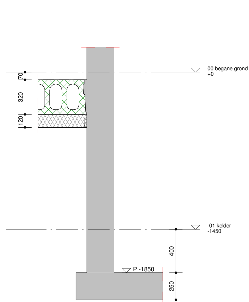
Detail 0.02 Schaal: 1 : 20
