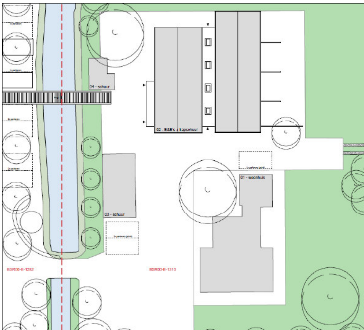
Figuur 2: Inrichtingsplan Zuiddijk 11 in Zuidoostbeemster
