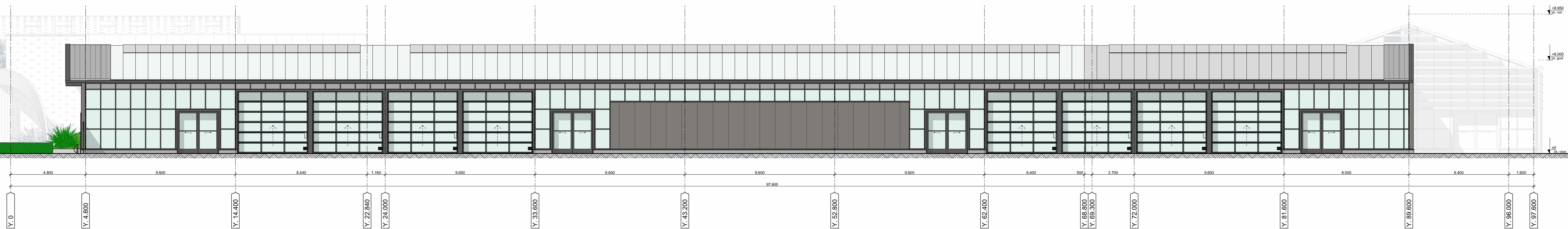
Rechtergevel - ZW Schaal 1:100
