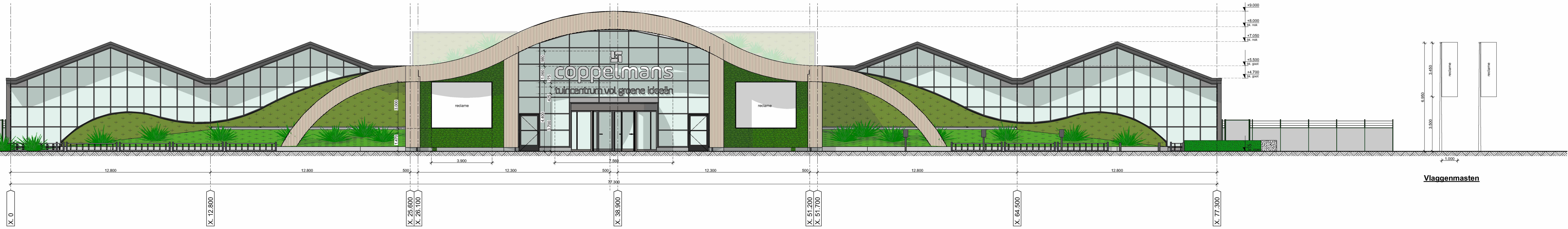
Voorgevel - NW Schaal 1:100
