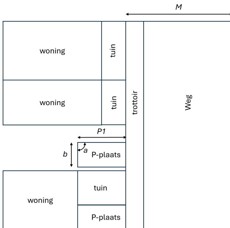
Figuur: Schematische weergave van opbouw van de totale lengte van de parkeereenheid
