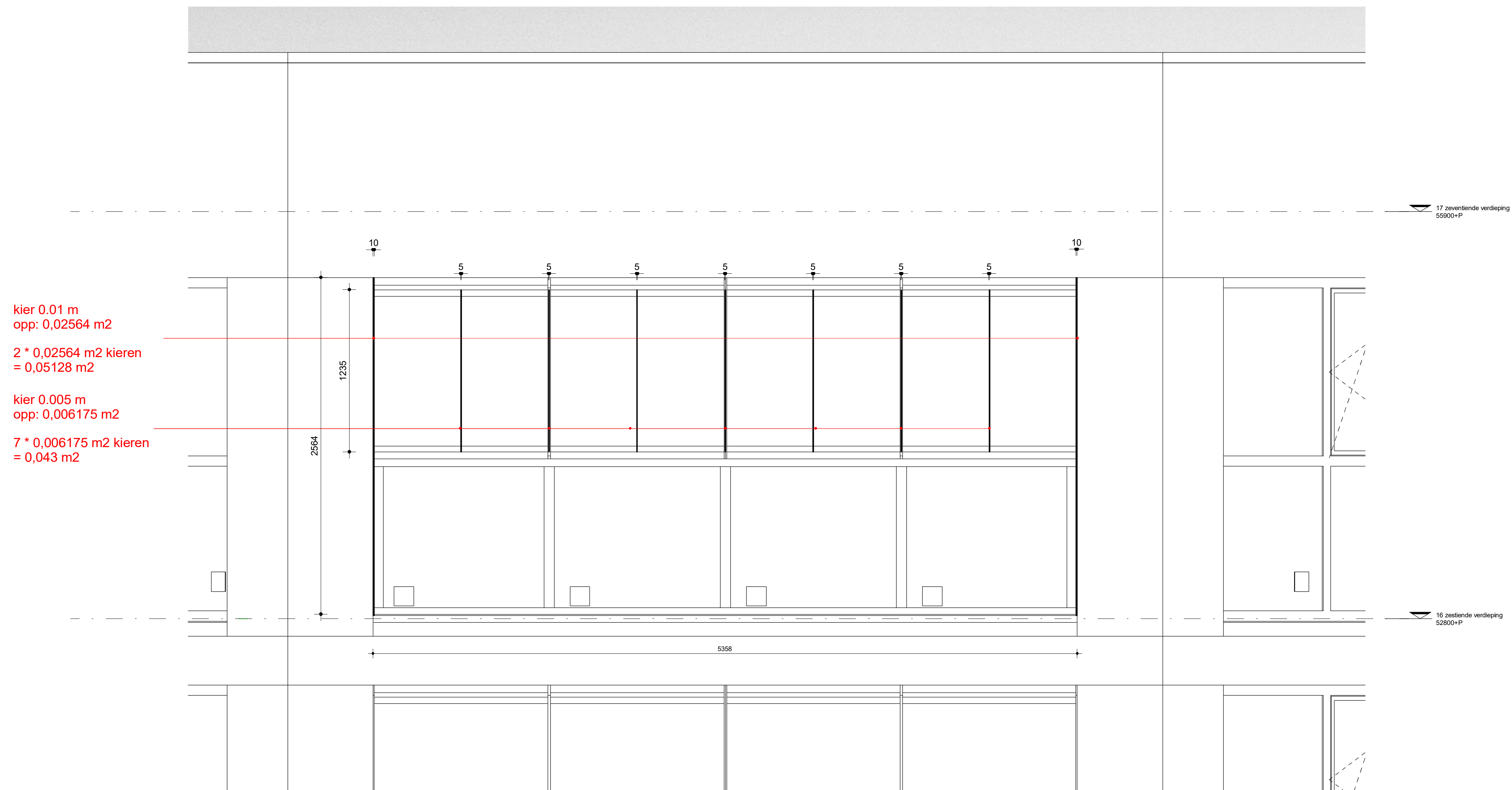
Aanzicht hoekwintertuin groot schaal 1 : 20
