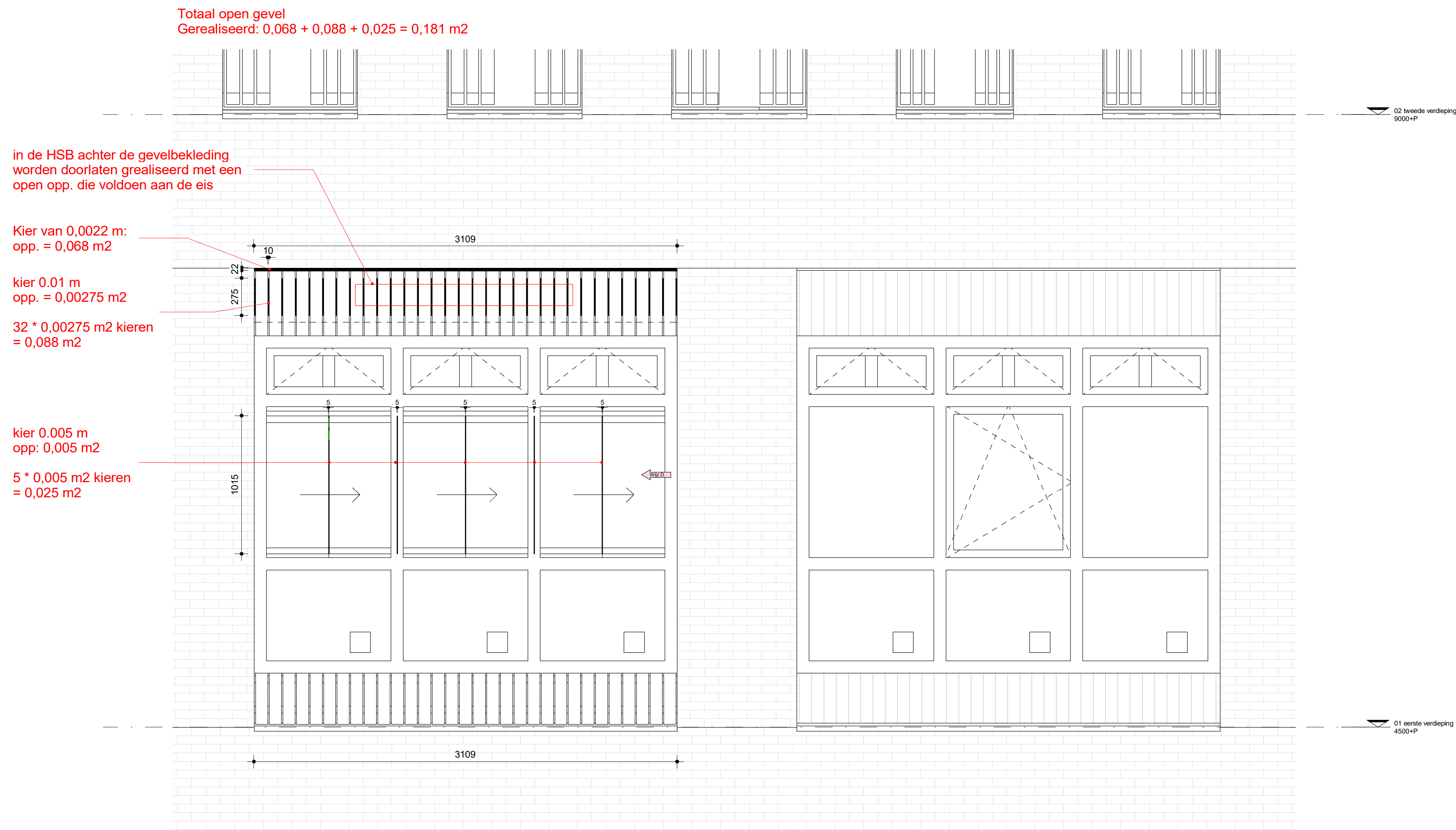
Zuidaanzicht Bnr. 1 schaal 1 : 20
