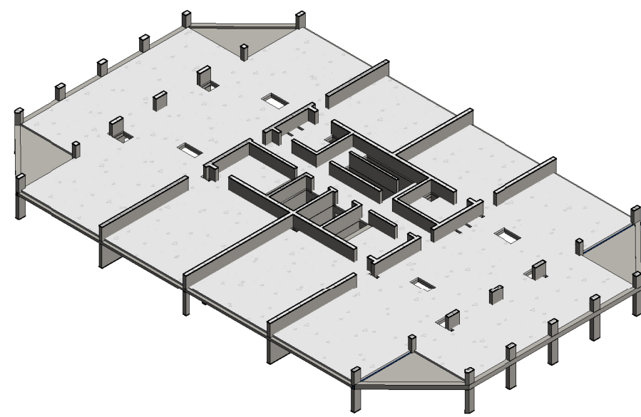
3D - 15e verdieping
