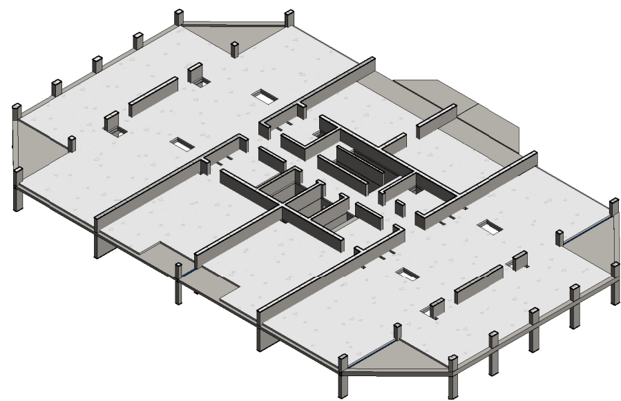
3D - 12e verdieping
