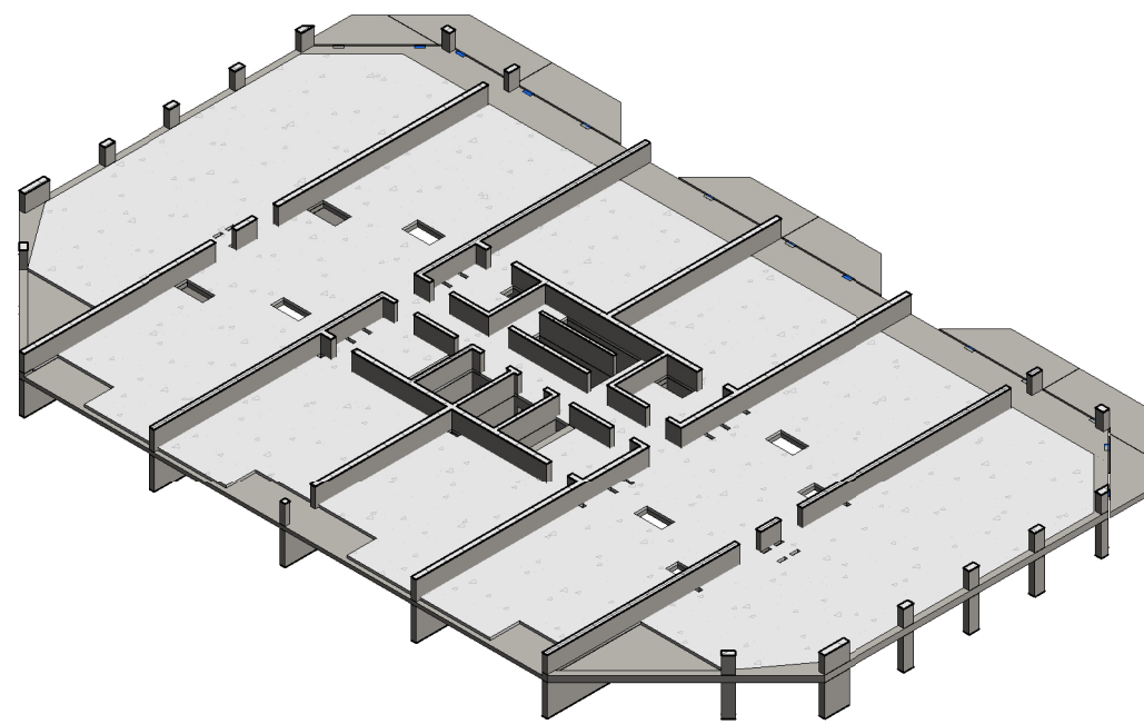
3D - 5e verdieping
