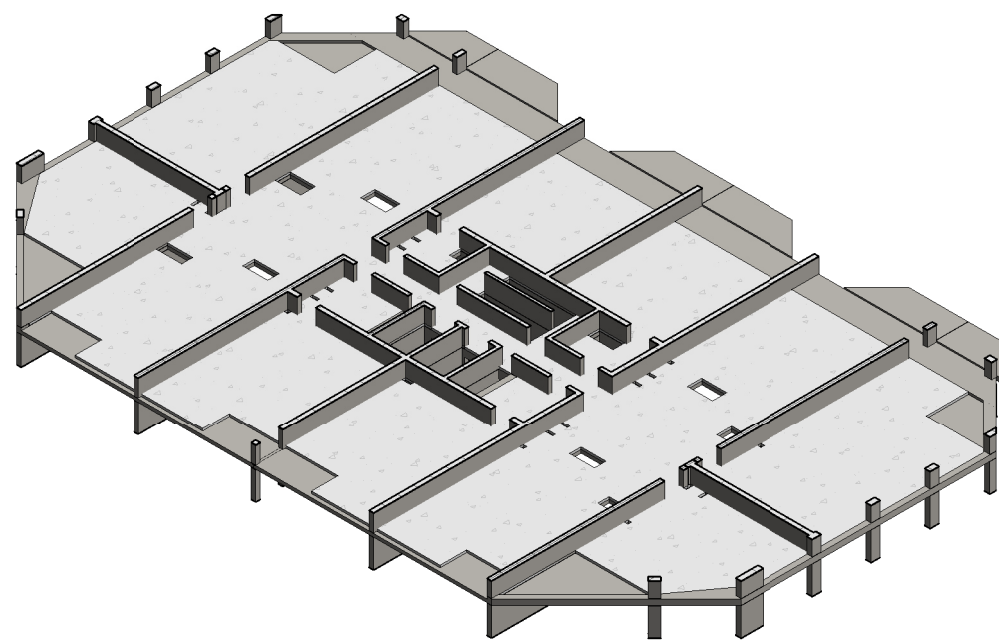
3D - 7e verdieping
