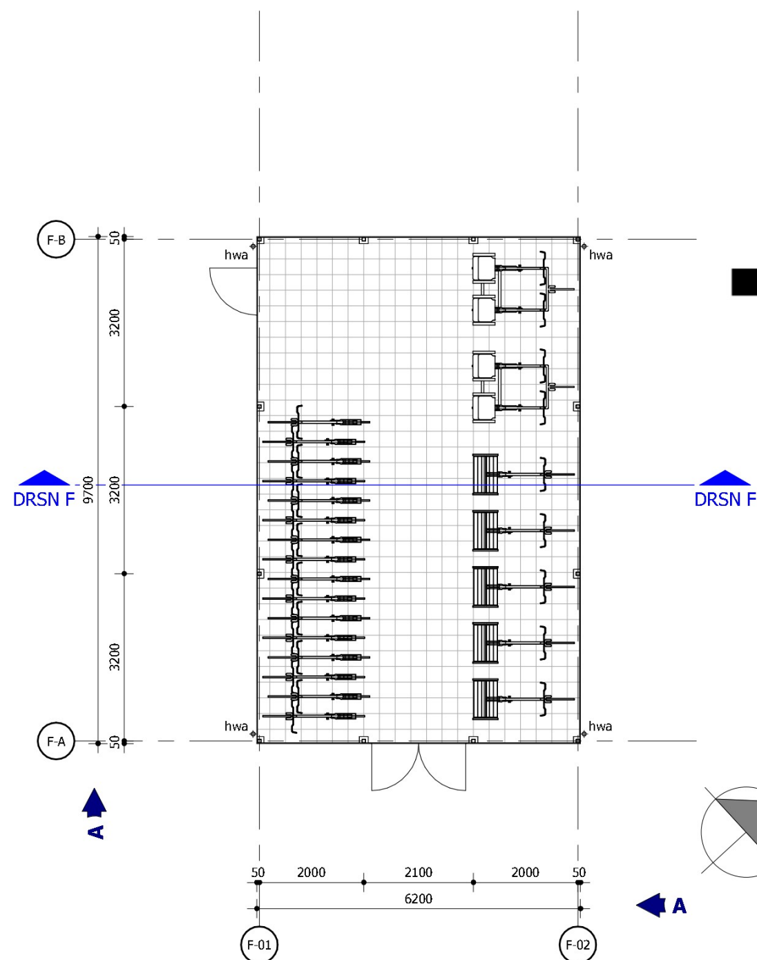
Plattegrond
