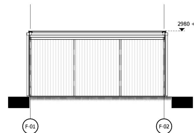
Doorsnede F-F
