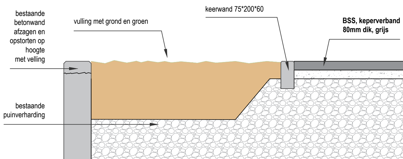
D01 doorsnede detail wijzigen inrit.
