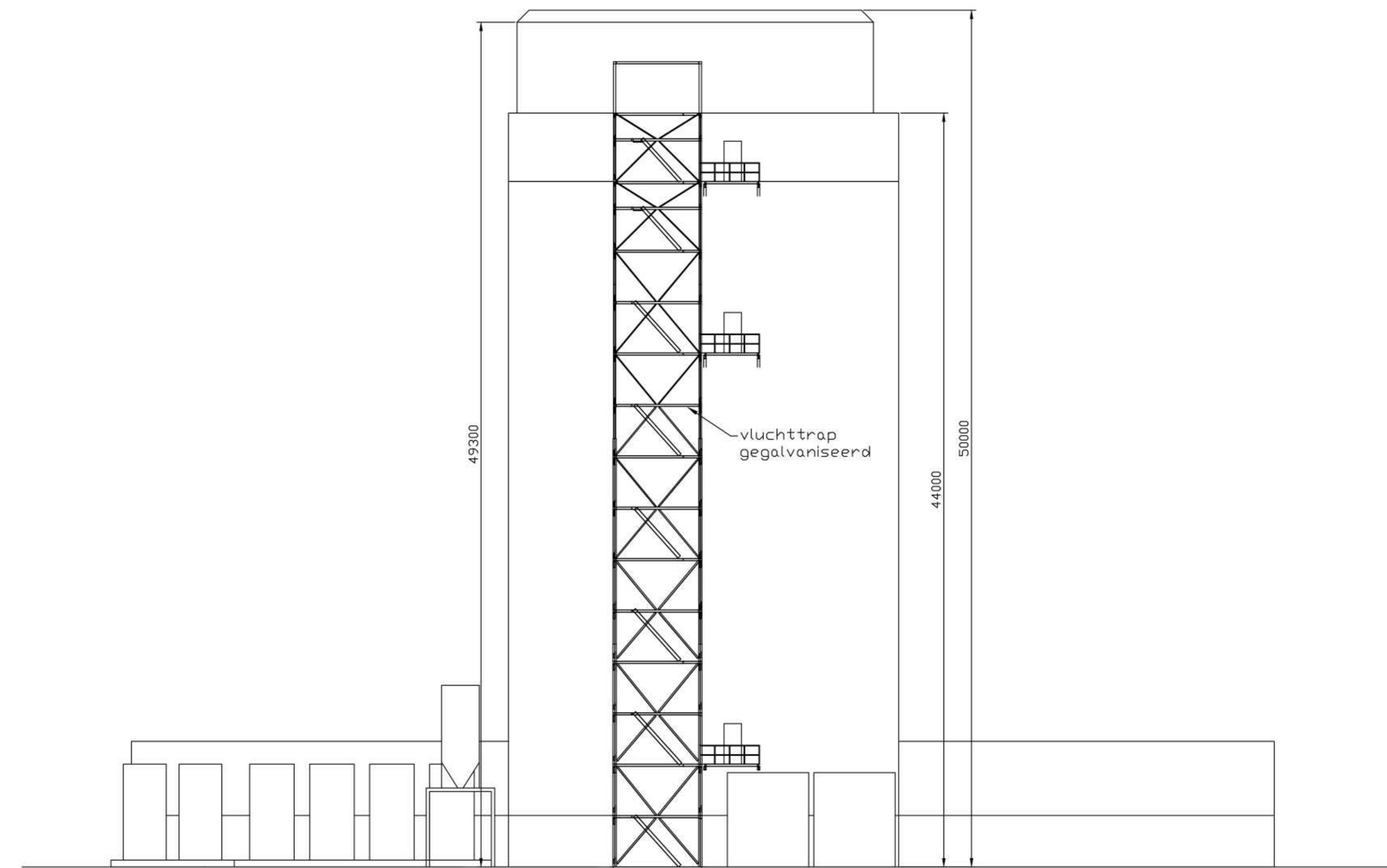
Zuidgevel
