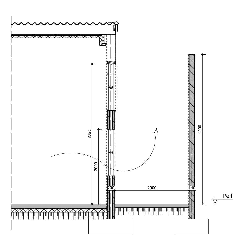
Doorsnede C Schaal 1:50 Doorsnede t.p.v. de stofbak stal 1
