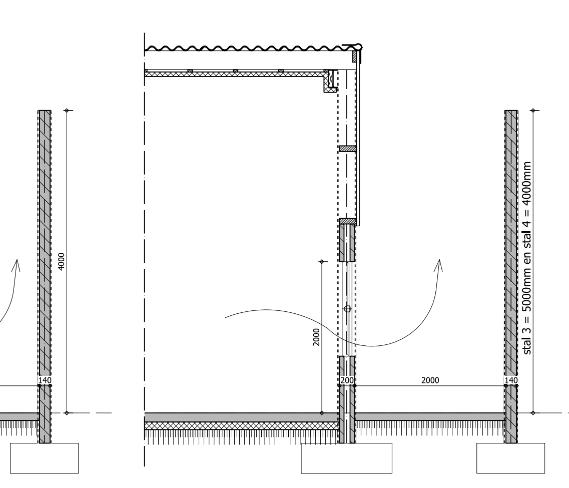
Doorsnede B Schaal 1:50 Doorsnede t.p.v. de stofbak stal 3 en 4
