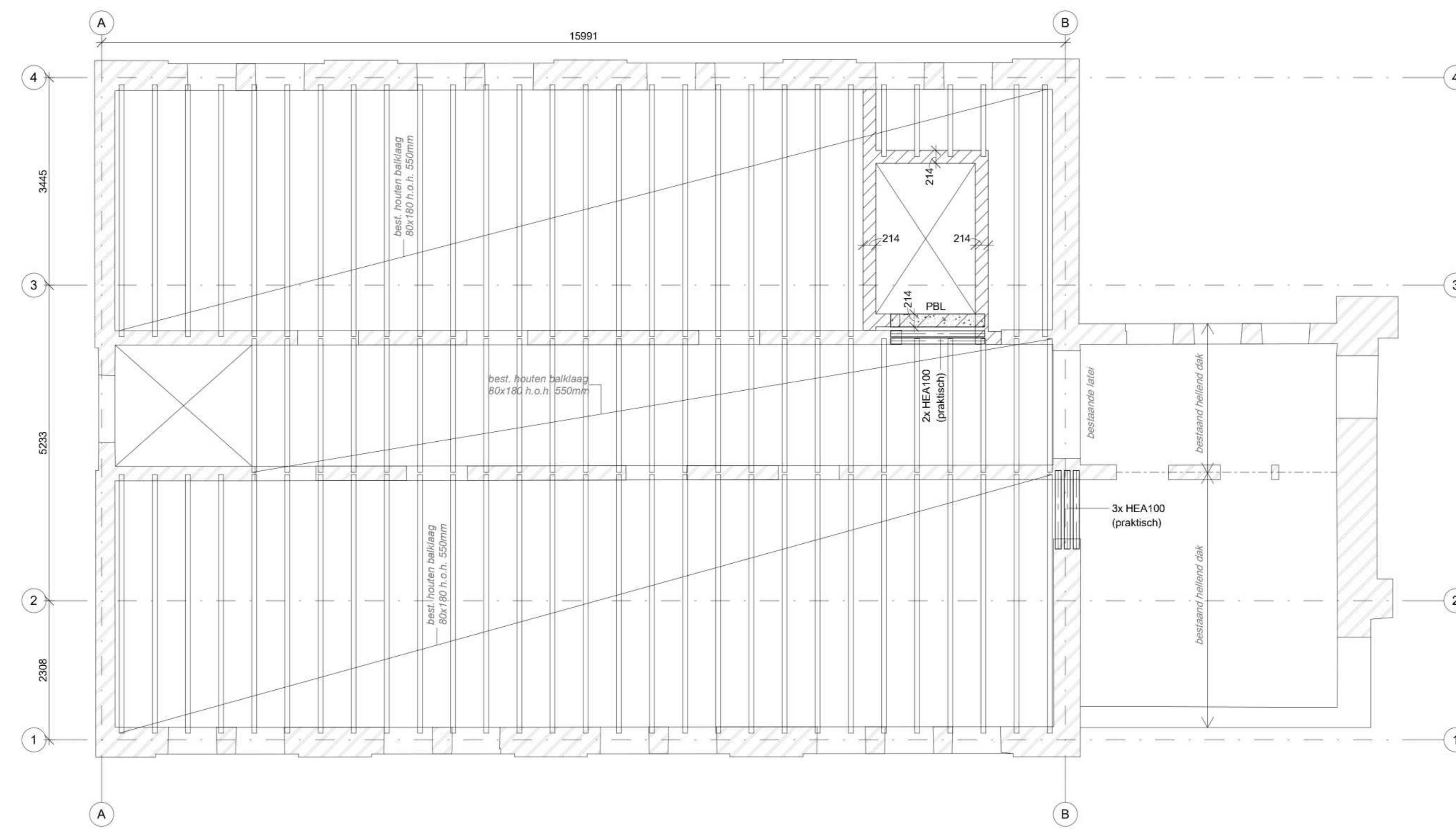
- 3e verdiepingsvloer - (schaal 1 : 50)
