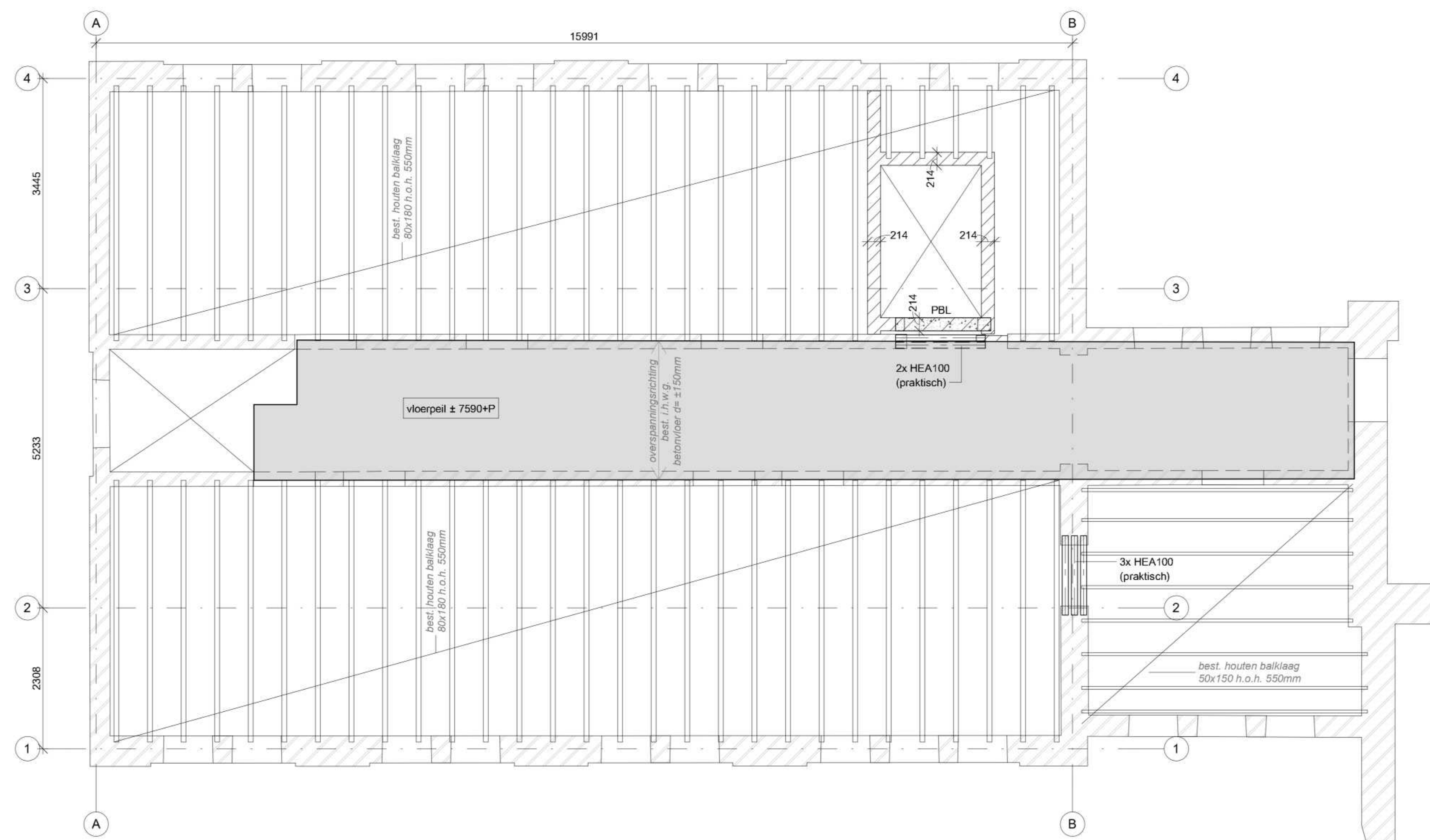
- 2e verdiepingsvloer - (schaal 1 : 50)
