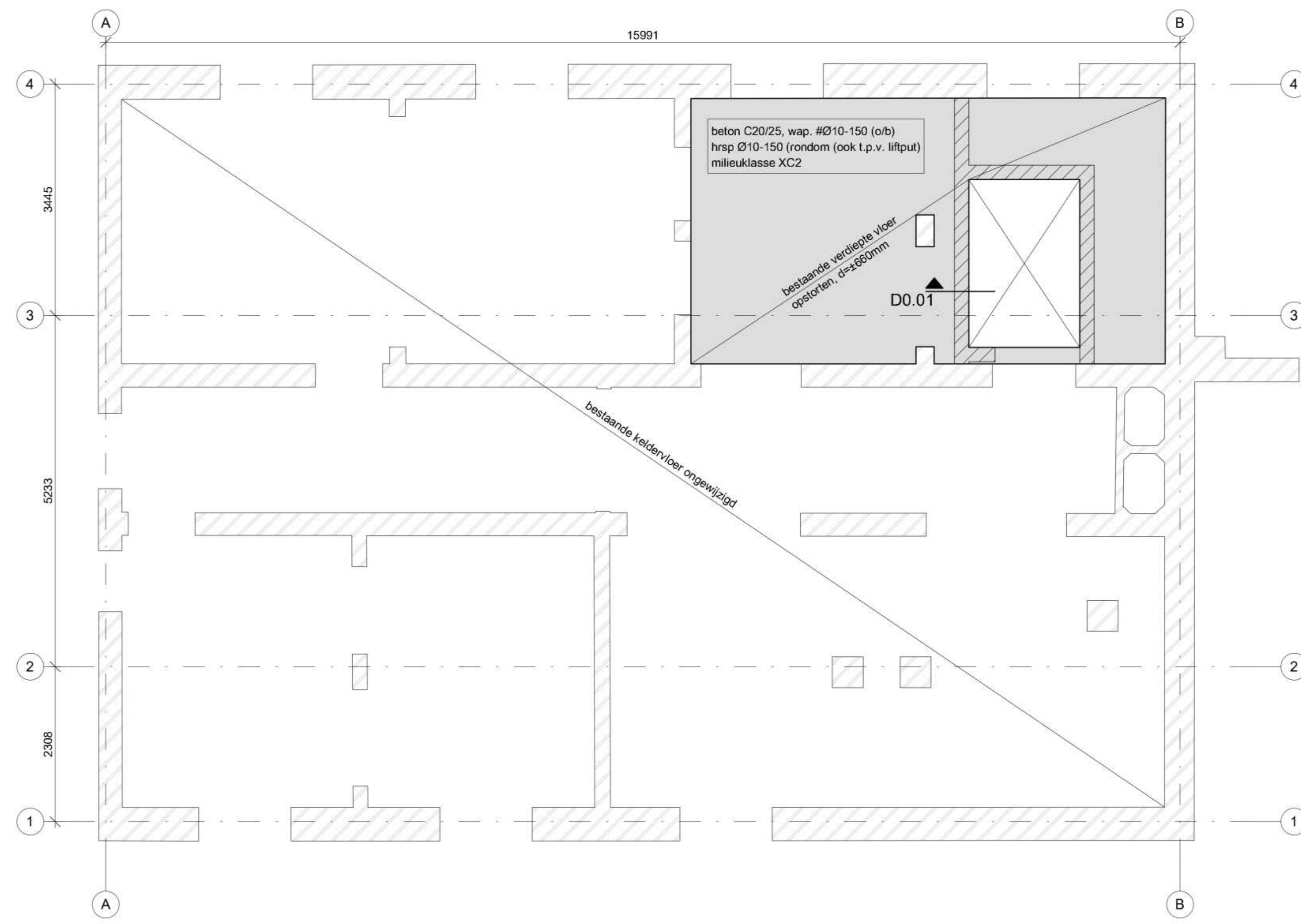
- keldervloer - (schaal 1 : 50)
