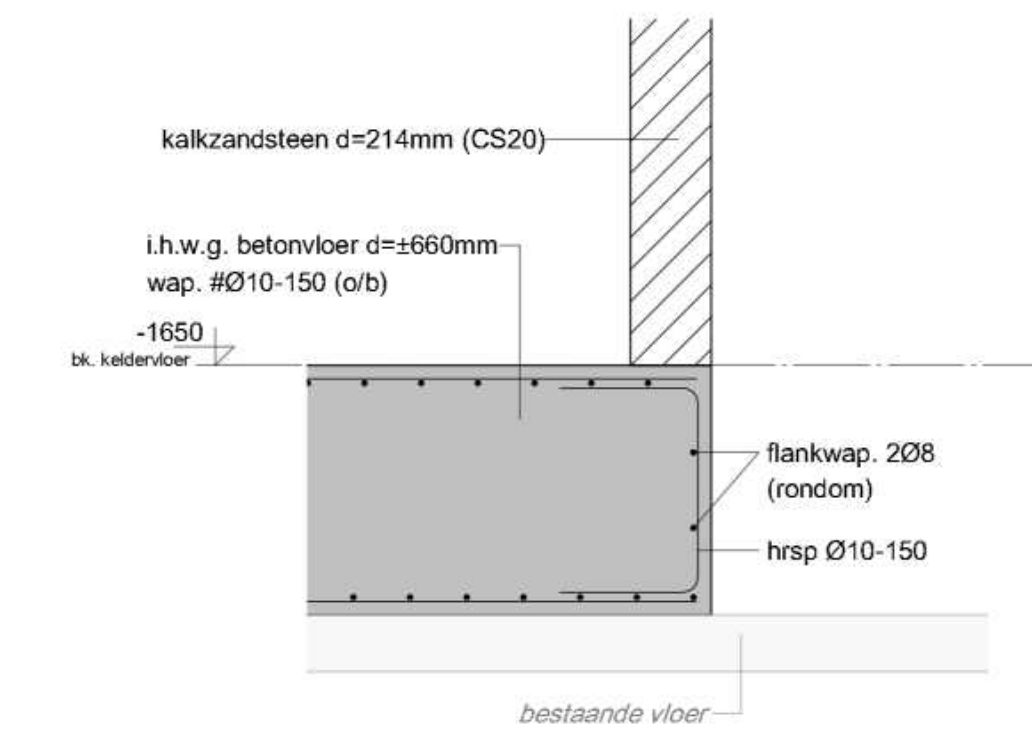
- D0.01 - (schaal 1 : 20)
