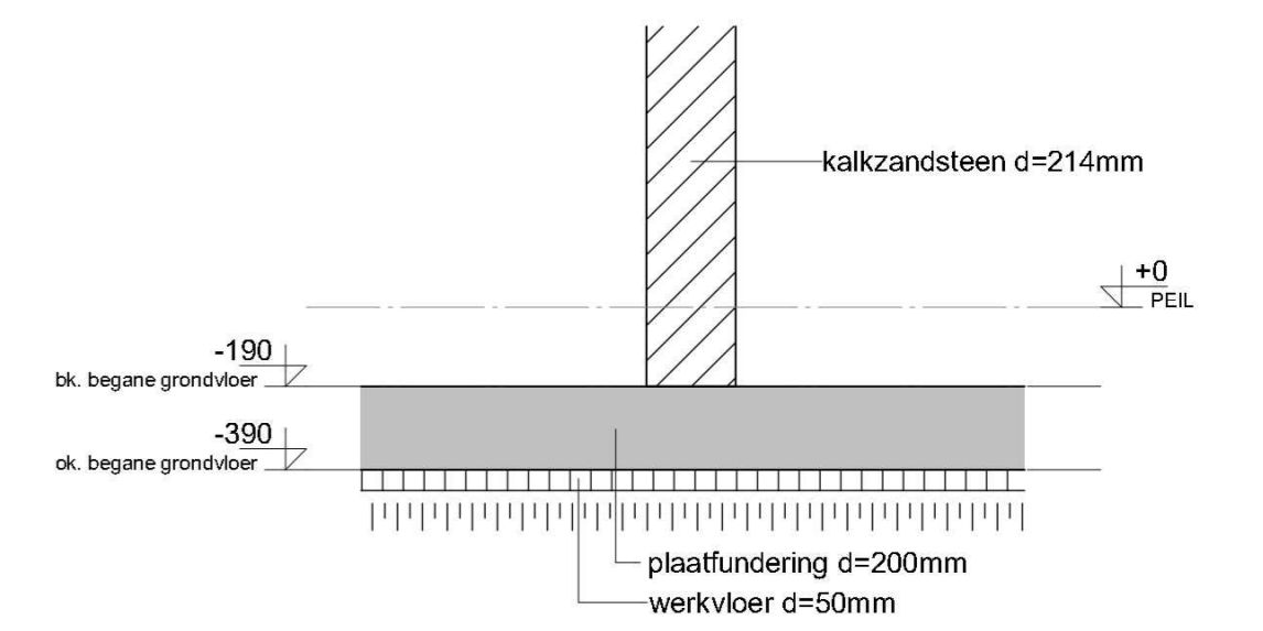
- D0.01 - (schaal 1 : 20)
