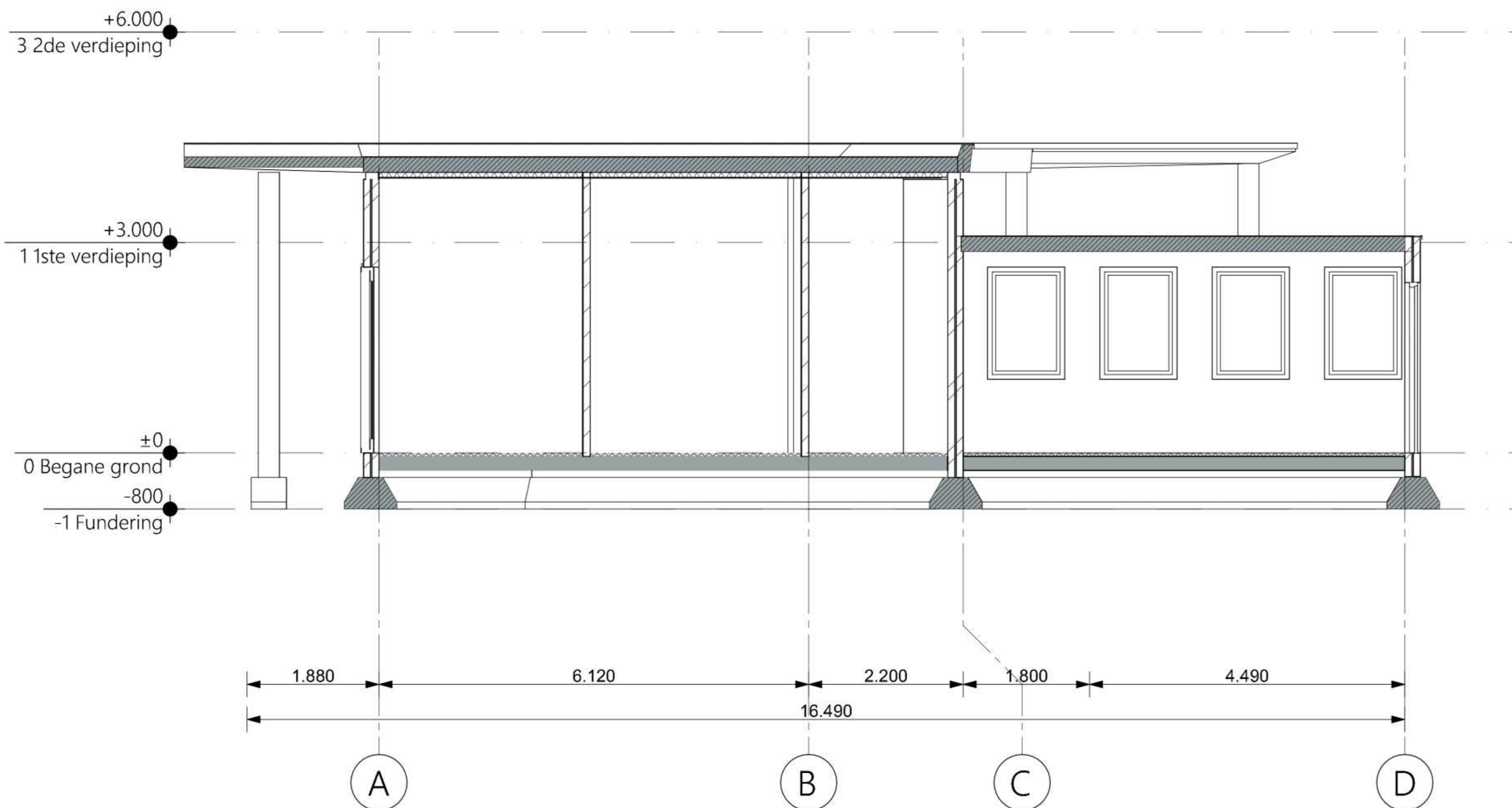
Doorsnede B-B bestaand - 1:50
