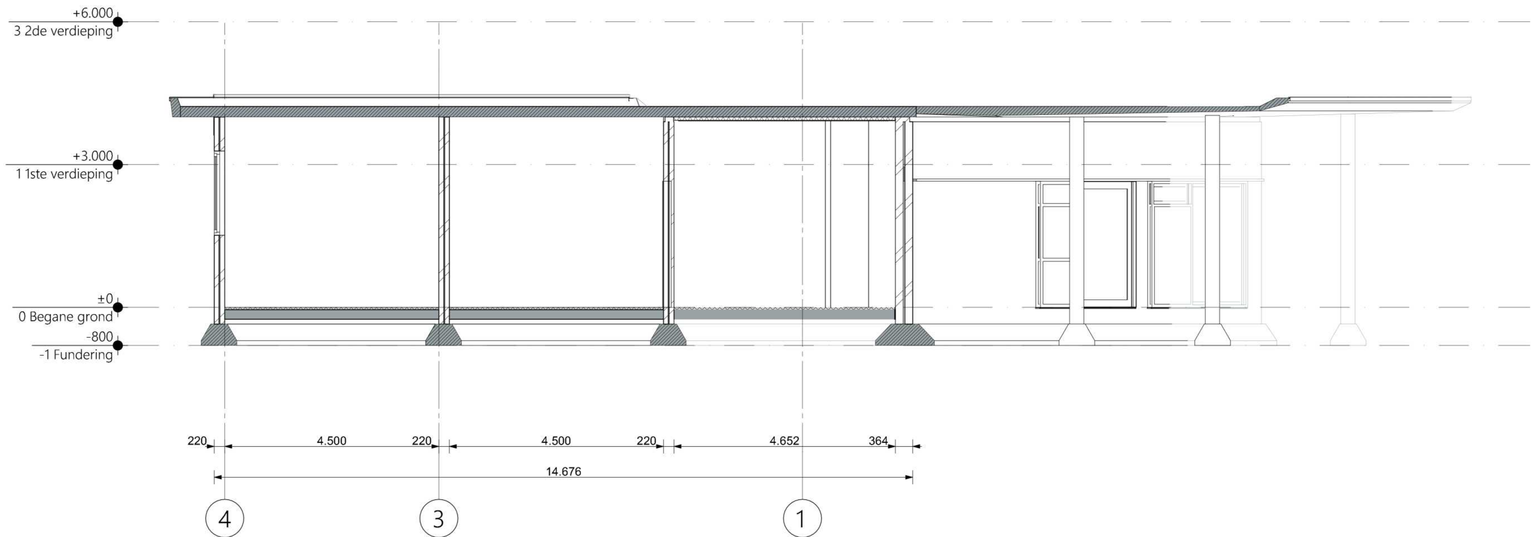
Doorsnede A-A bestaand - 1:50
