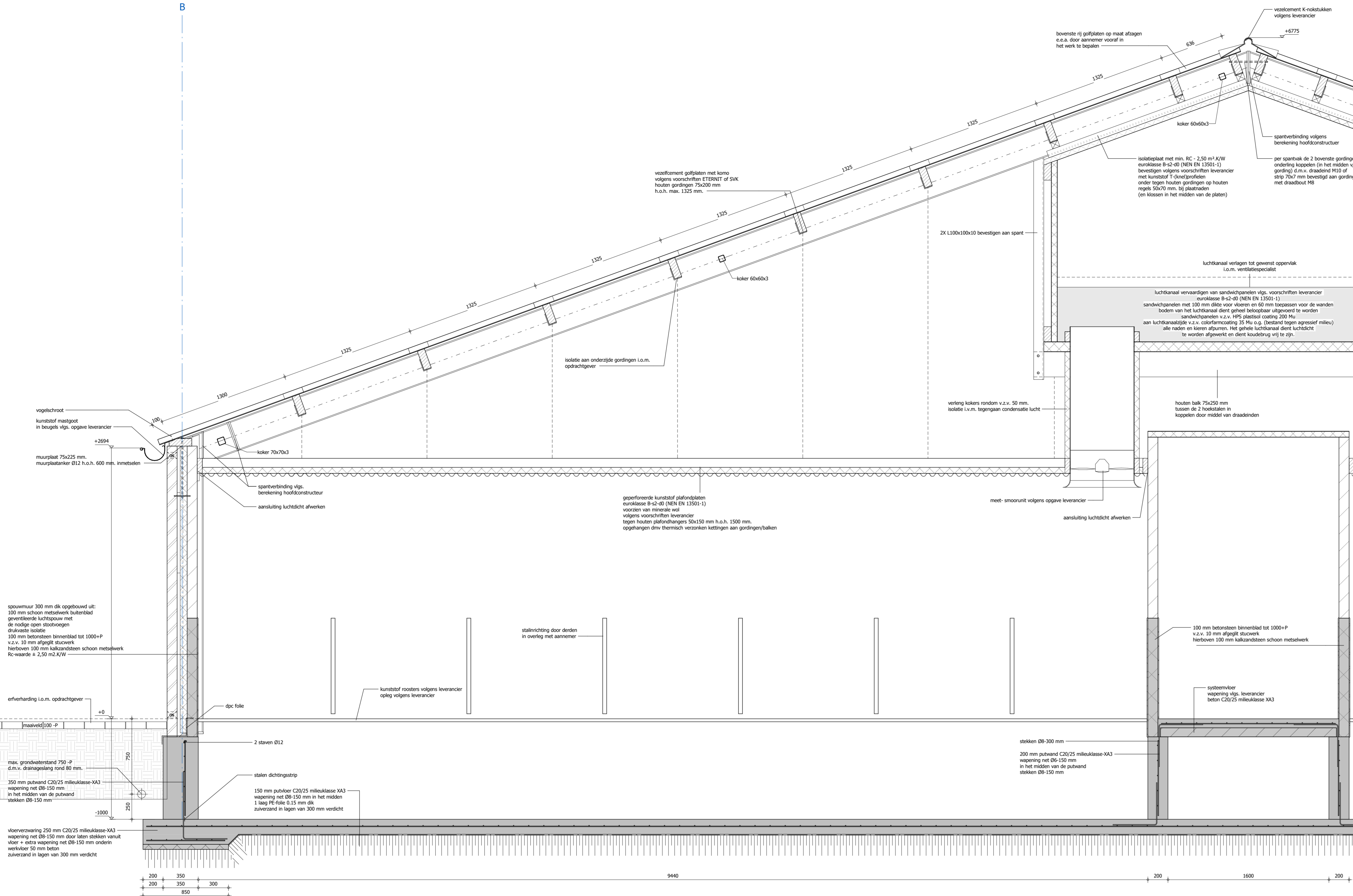
DOORSNEDE A-A
