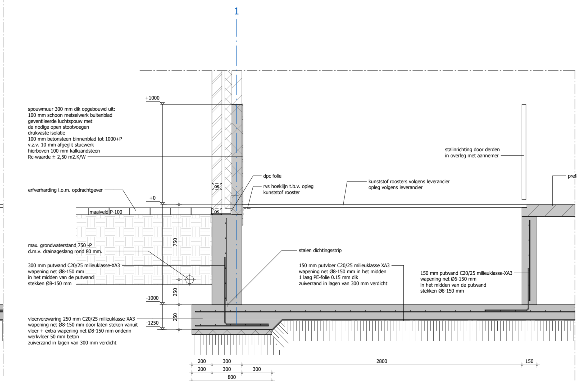
DOORSNEDE B-B
