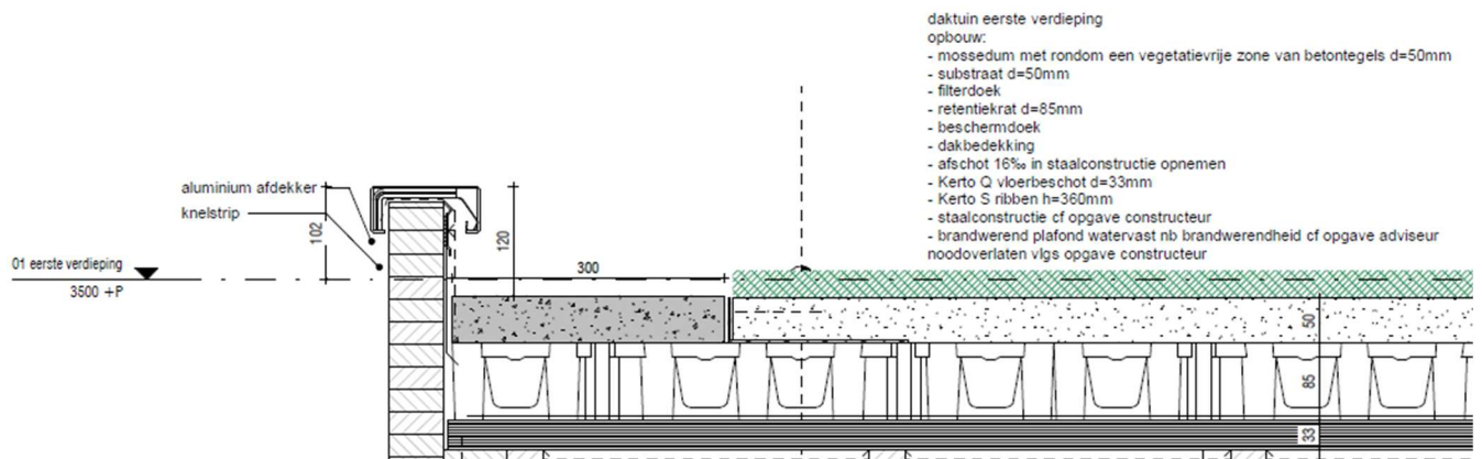
Randdetail groendak o.b.v. bouwkundig detail D210.
