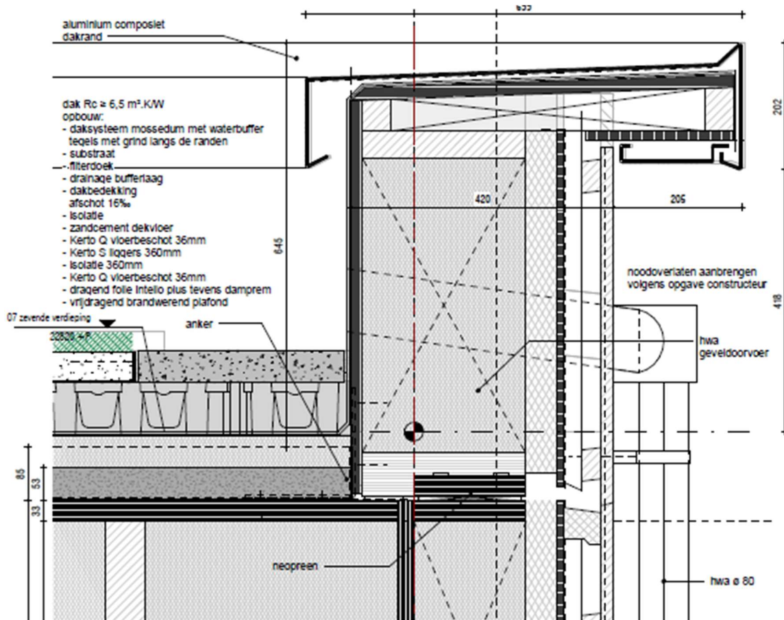
Randdetail groendak o.b.v. bouwkundig detail D304.
