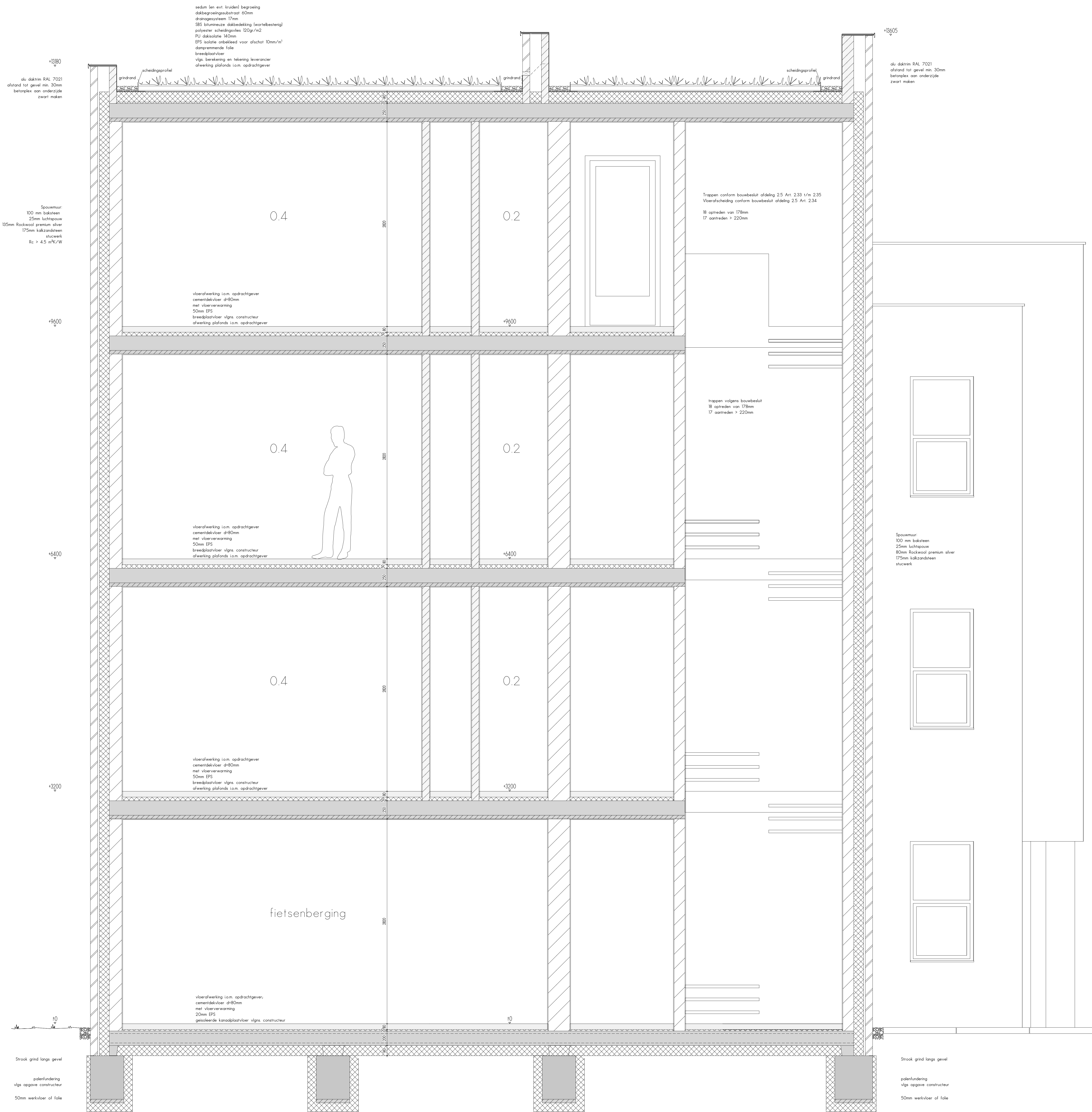
DOORSNEDE E
