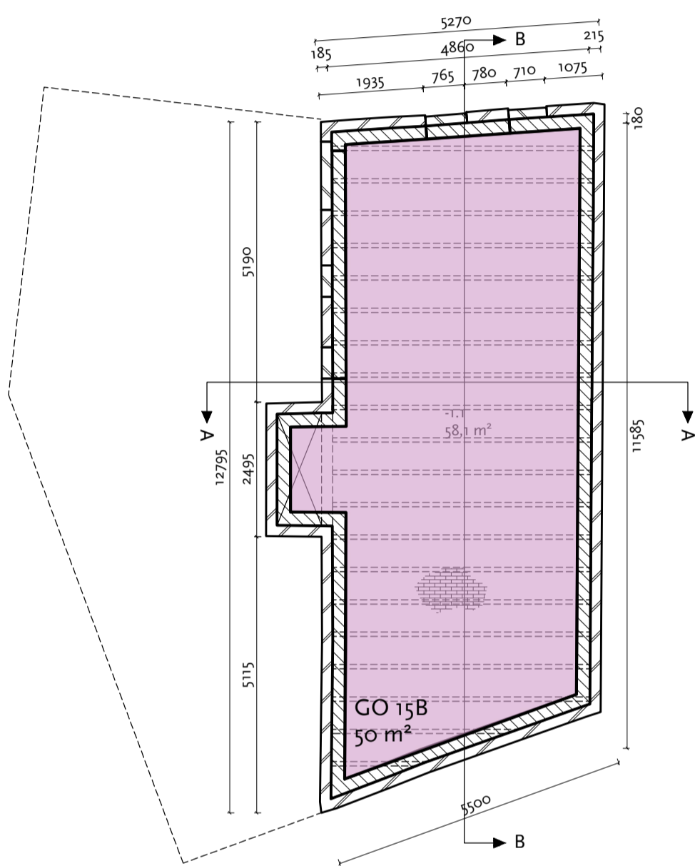
souterrain
