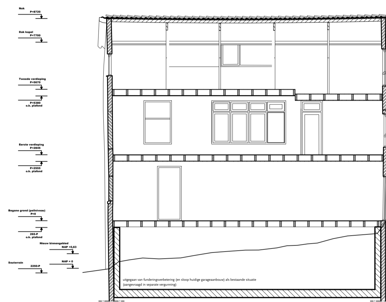
Doorsnede B-B
