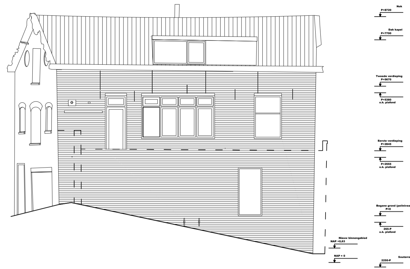
rechter zijgevel
