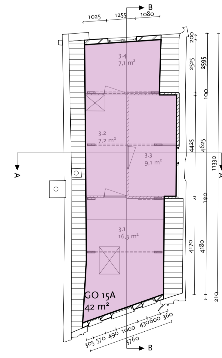
tweede verdieping
