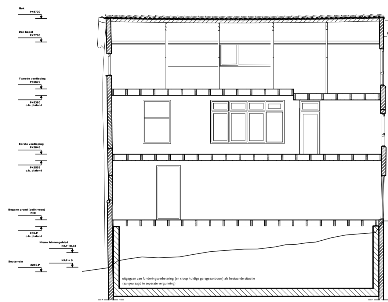
Doorsnede B-B
