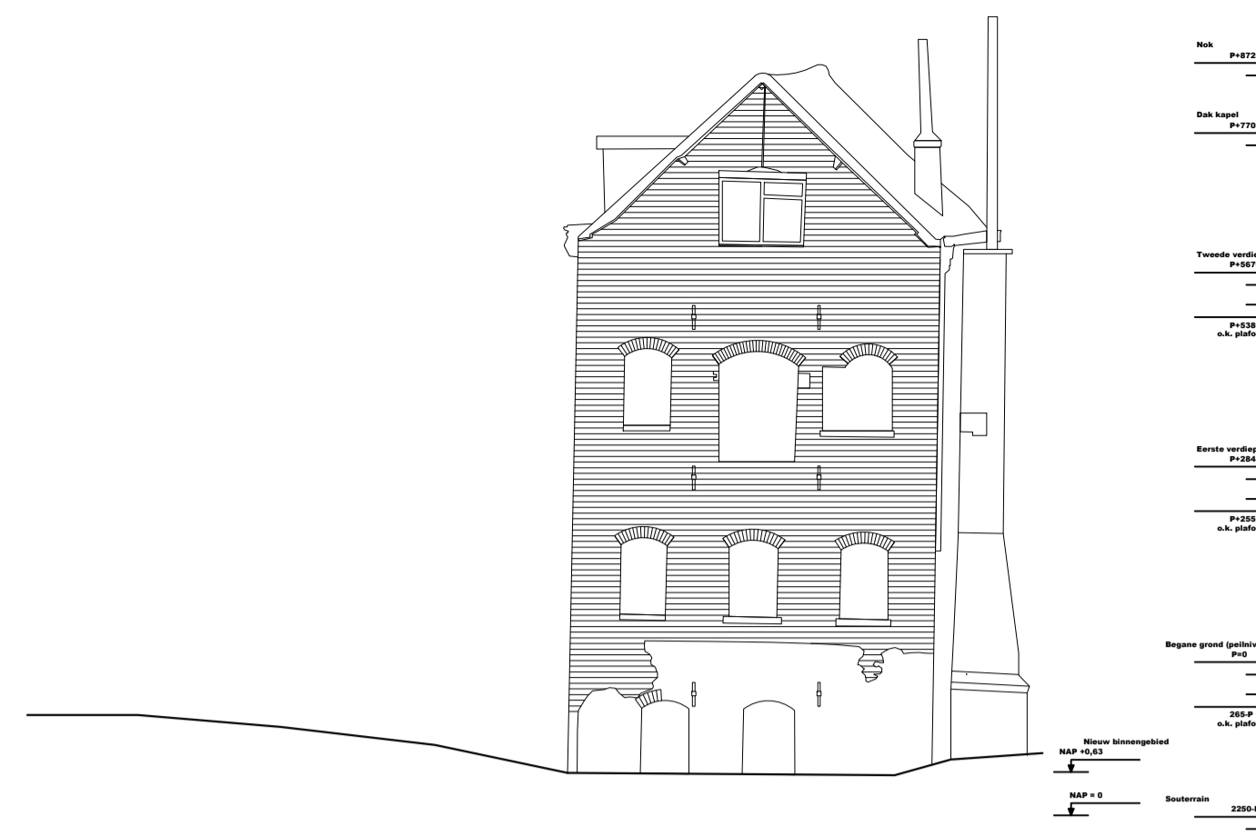
achtergevel
