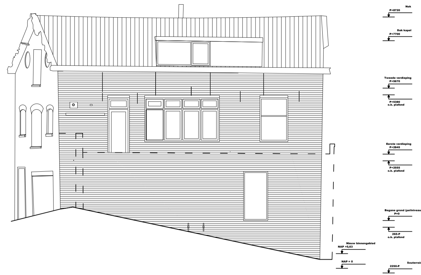
rechter zijgevel
