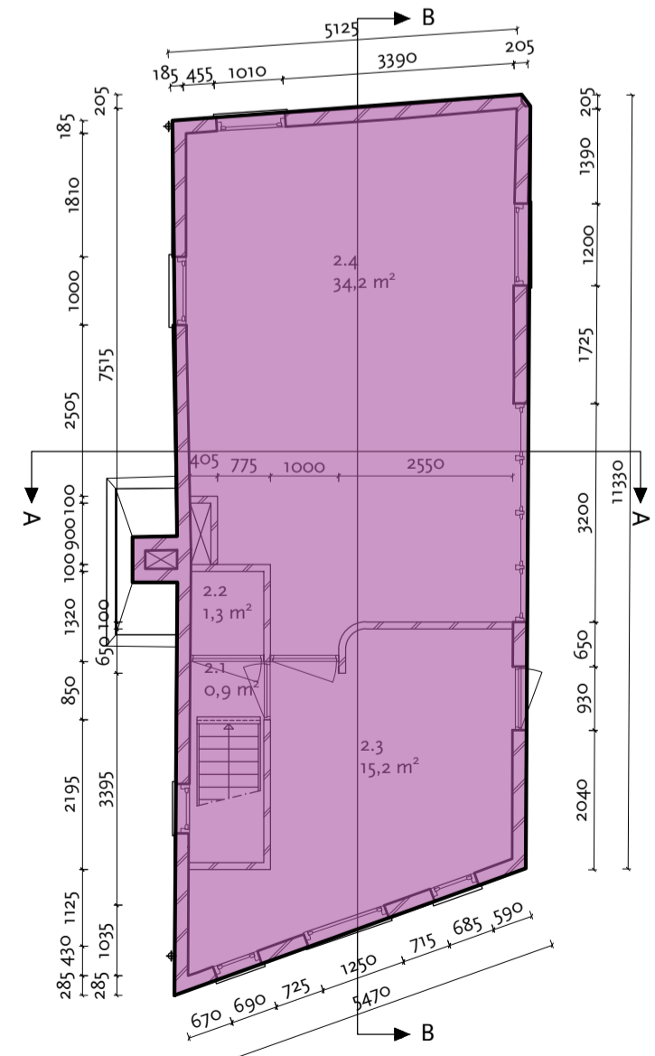
eerste verdieping
