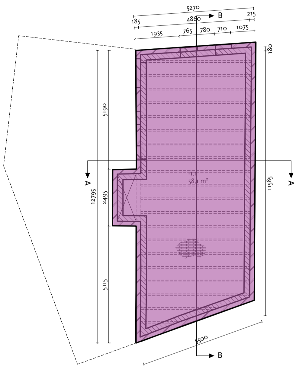
souterrain
