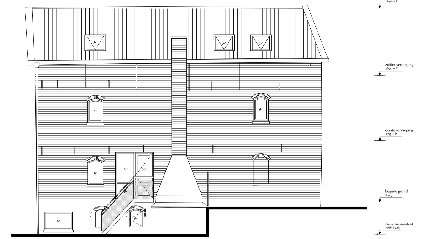
linker zijgevel
