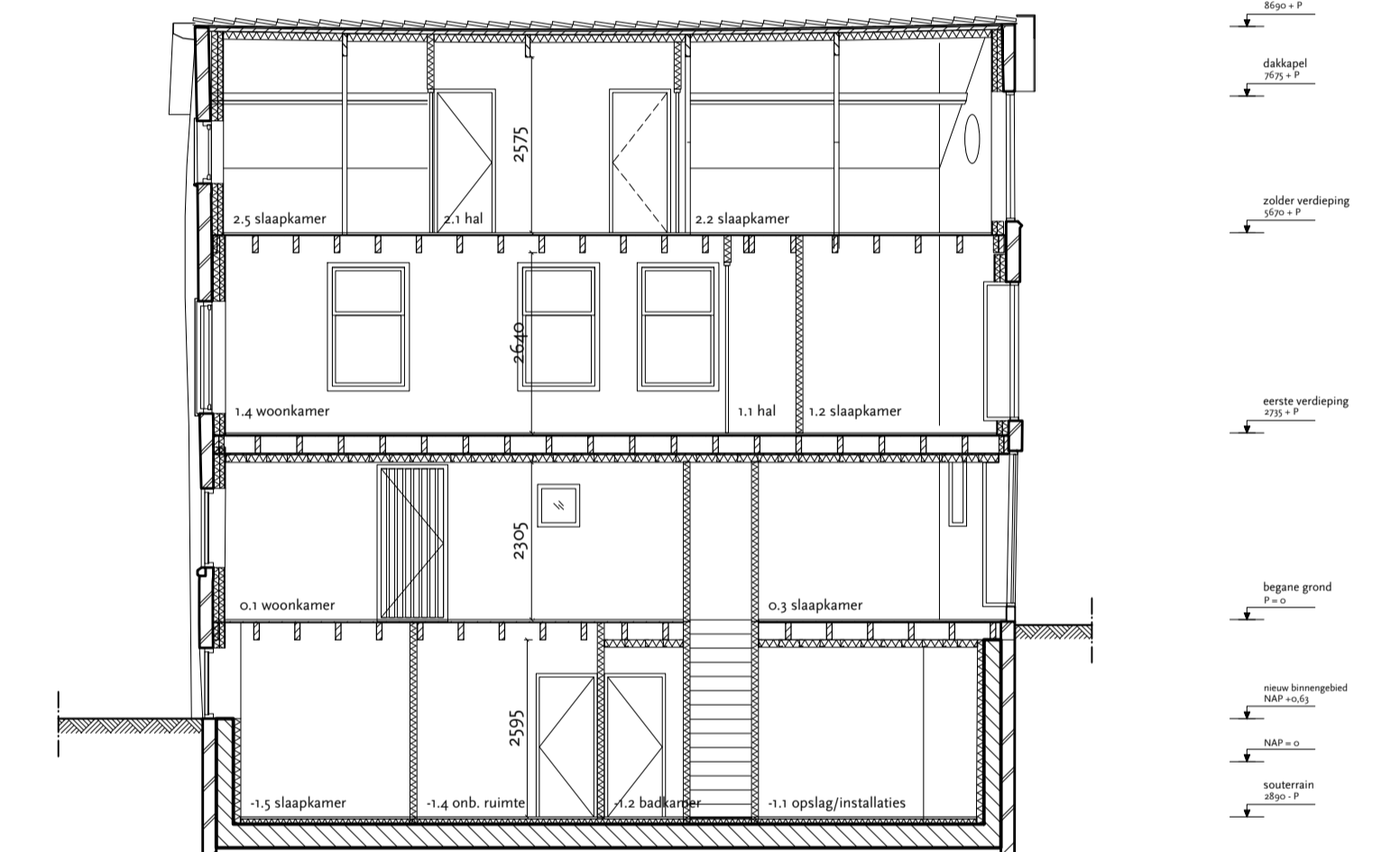
Doorsnede B-B
