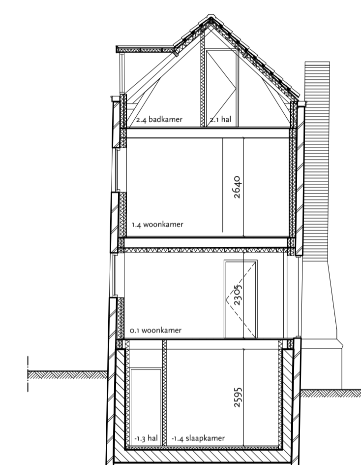
Doorsnede A-A
