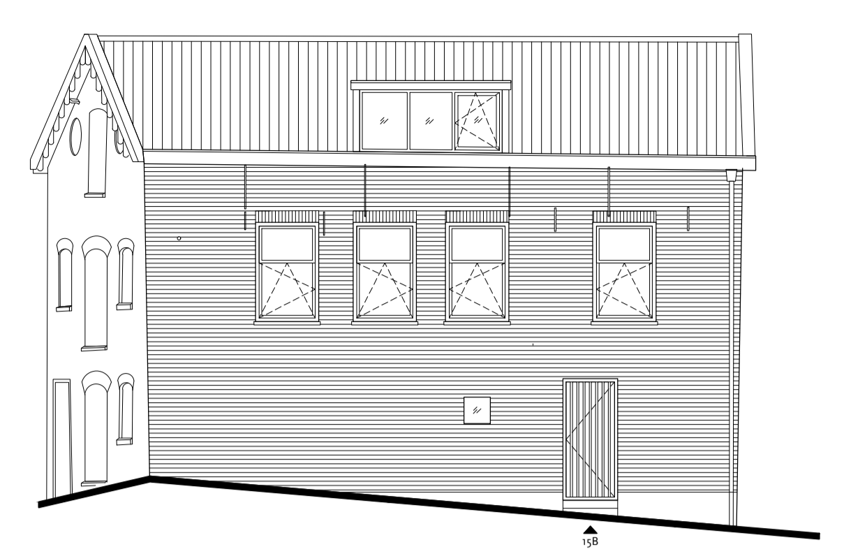
rechter zijgevel
