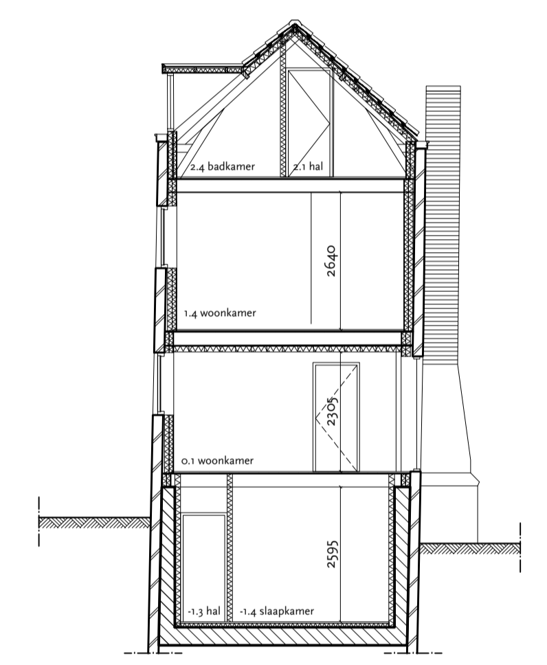
Doorsnede A-A
