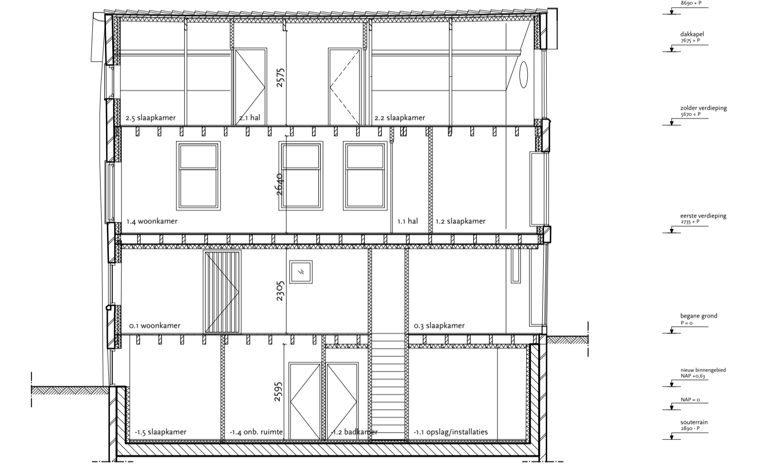
Doorsnede B-B
