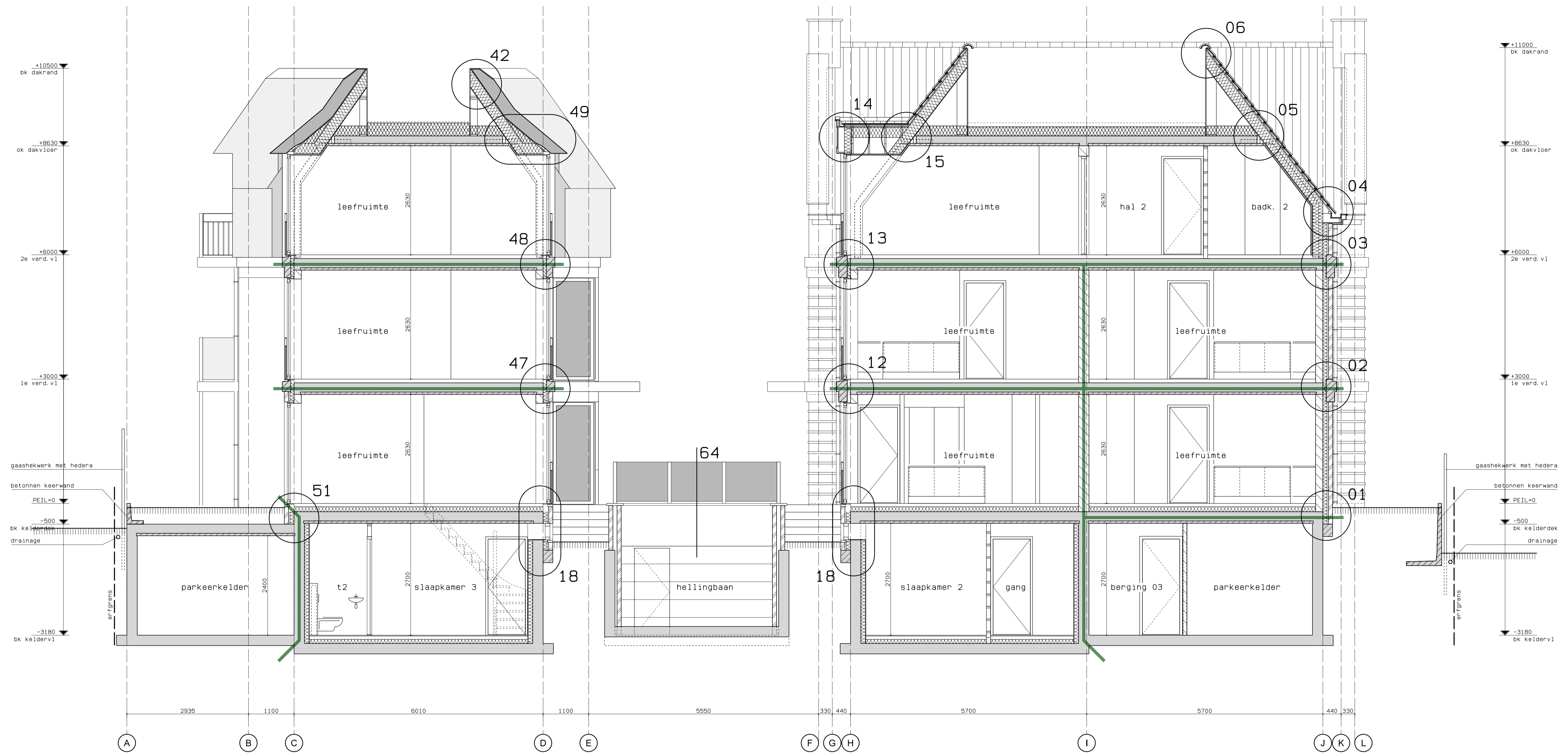
doorsnede E-E
