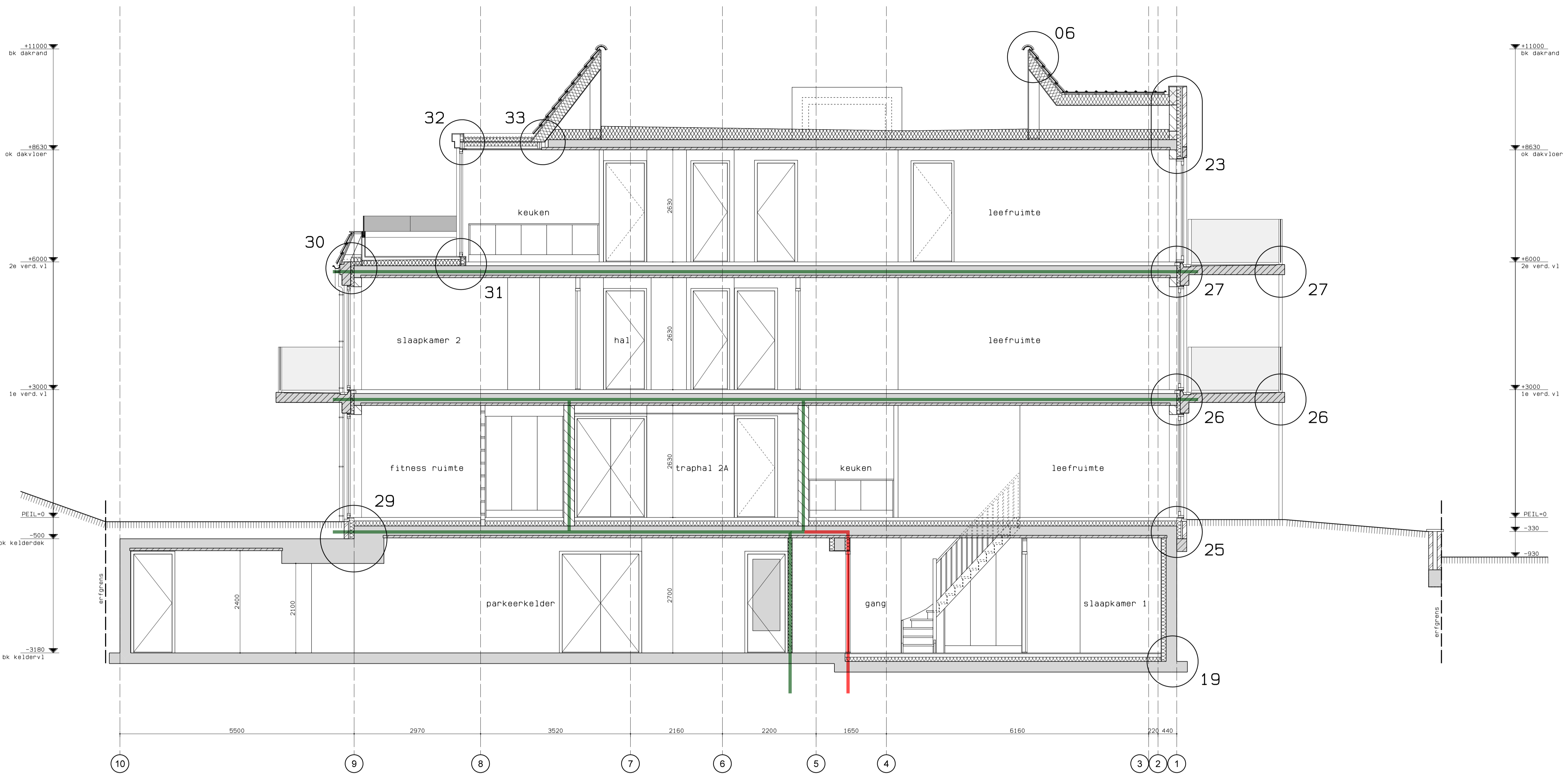
doorsnede D-D
