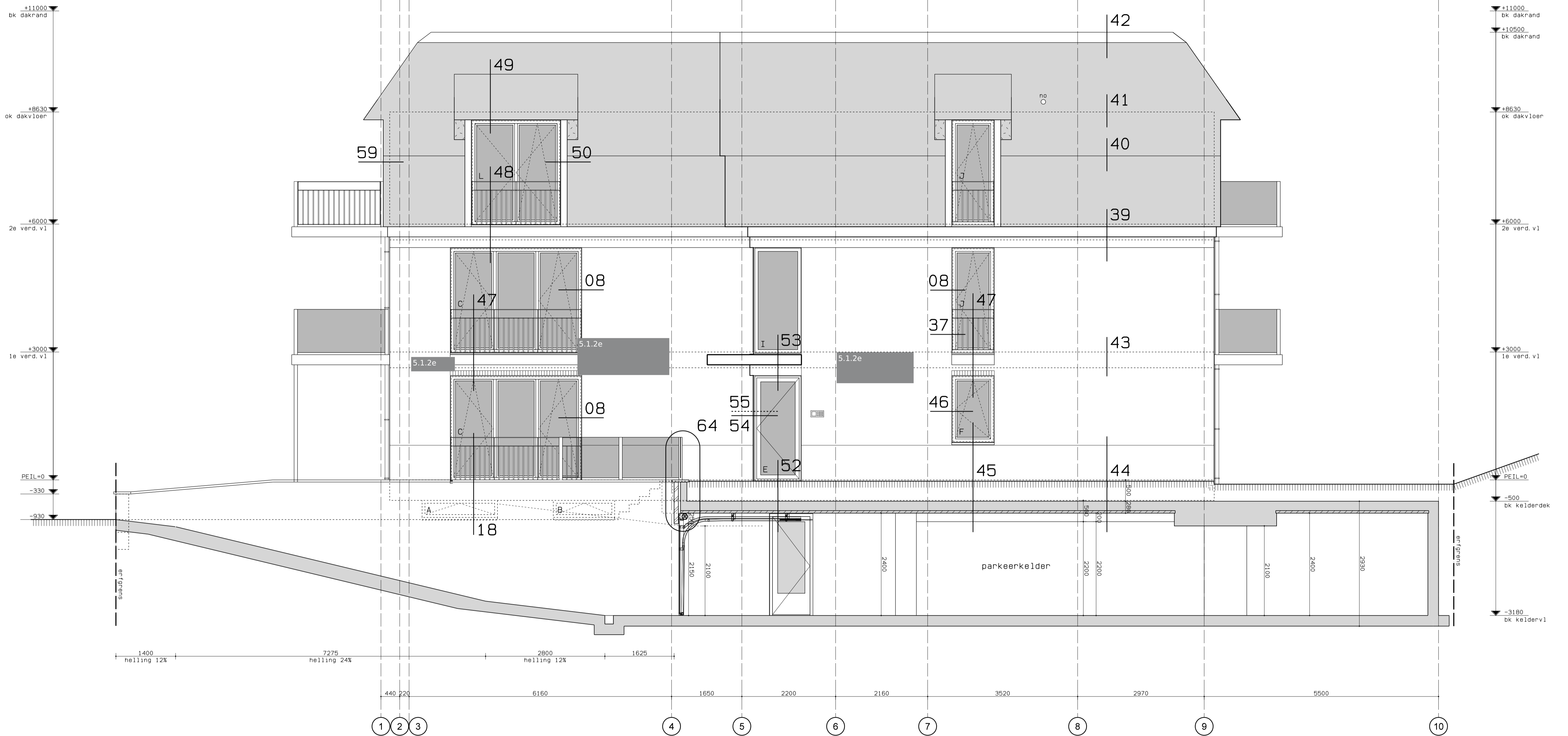
doorsnede B-B
