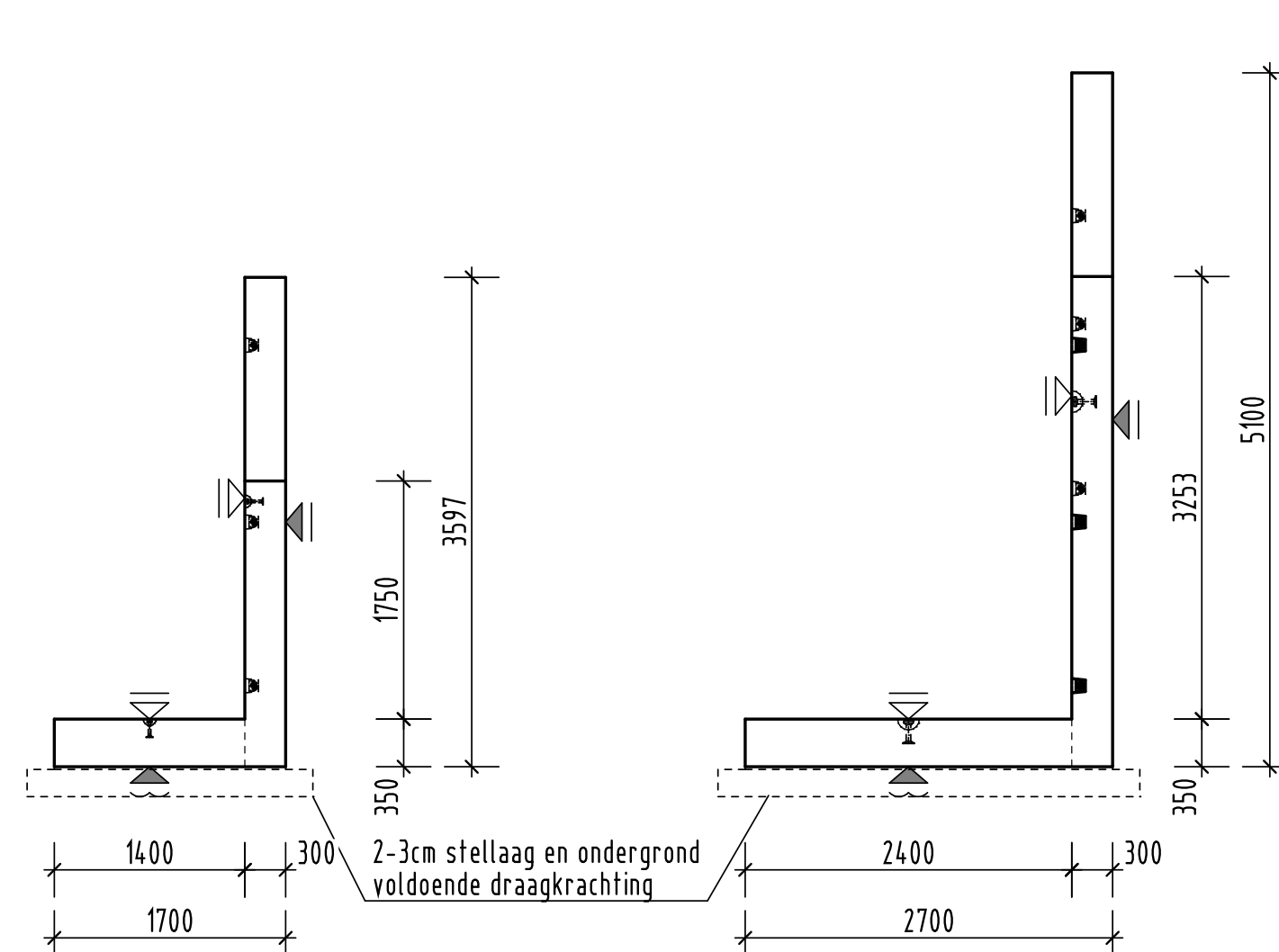
doorsnede C-C
