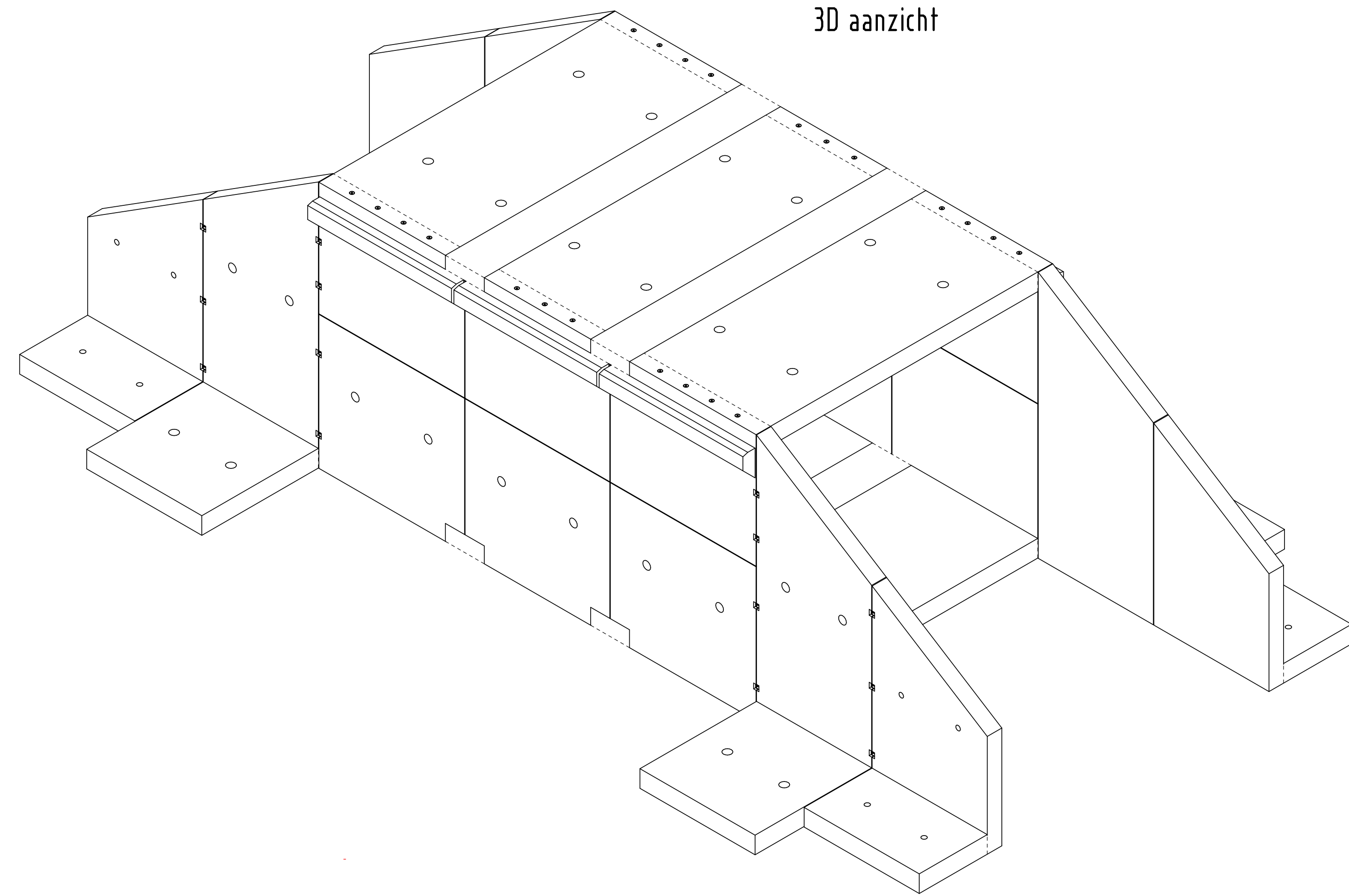
3D aanzicht
