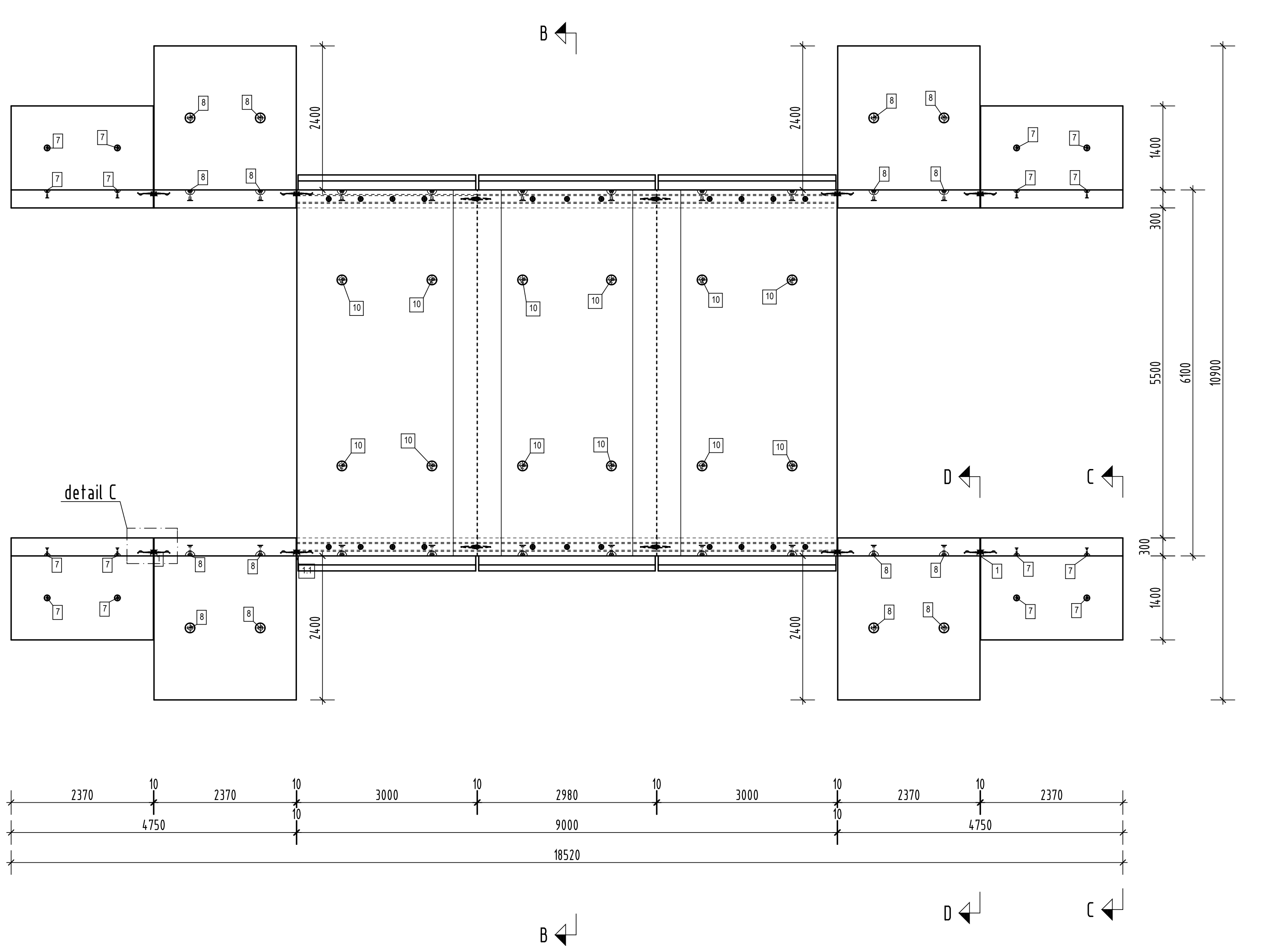
bovenaanzicht
