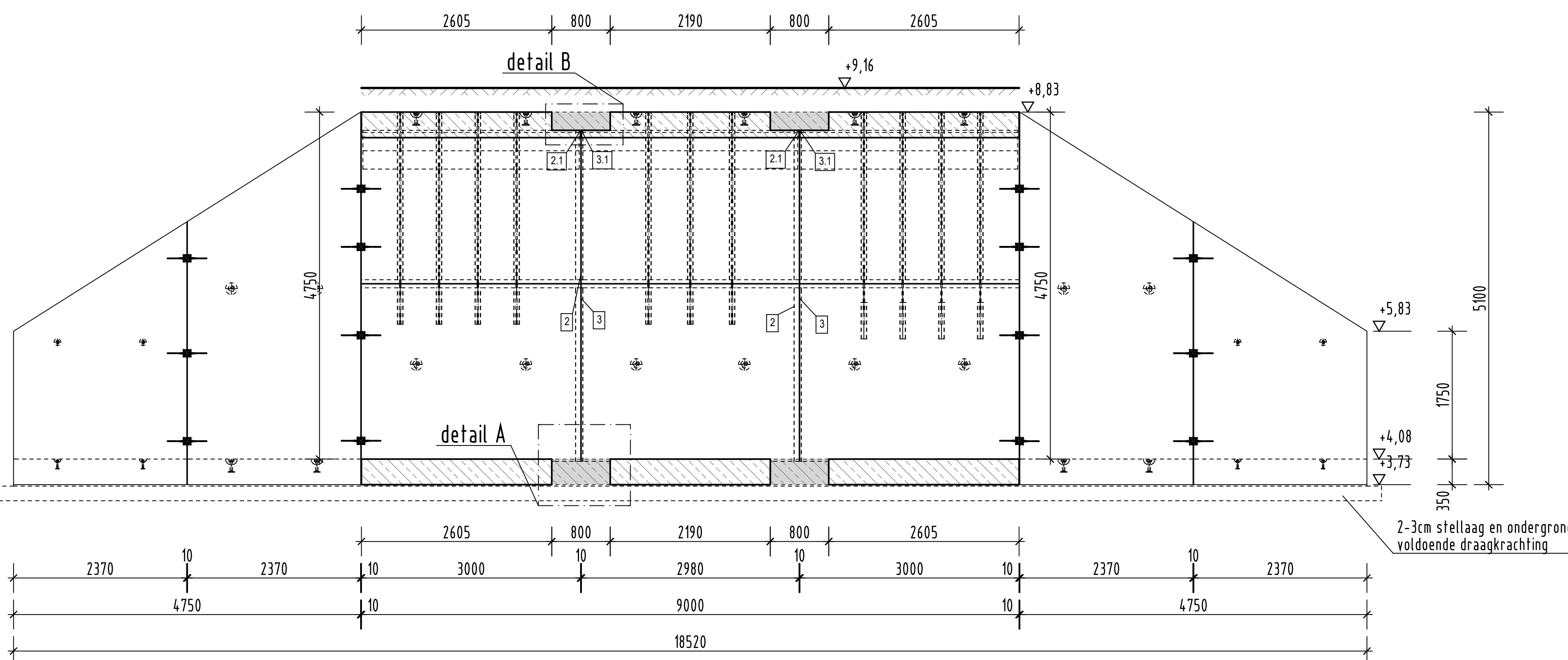
doorsnede A-A
