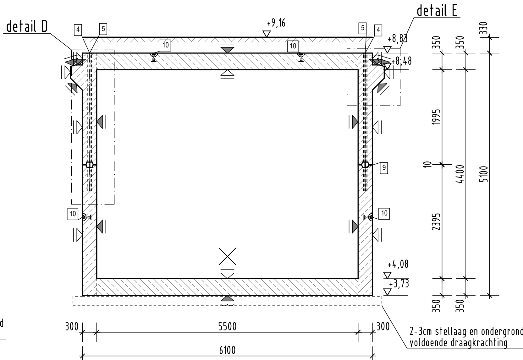
doorsnede B-B
