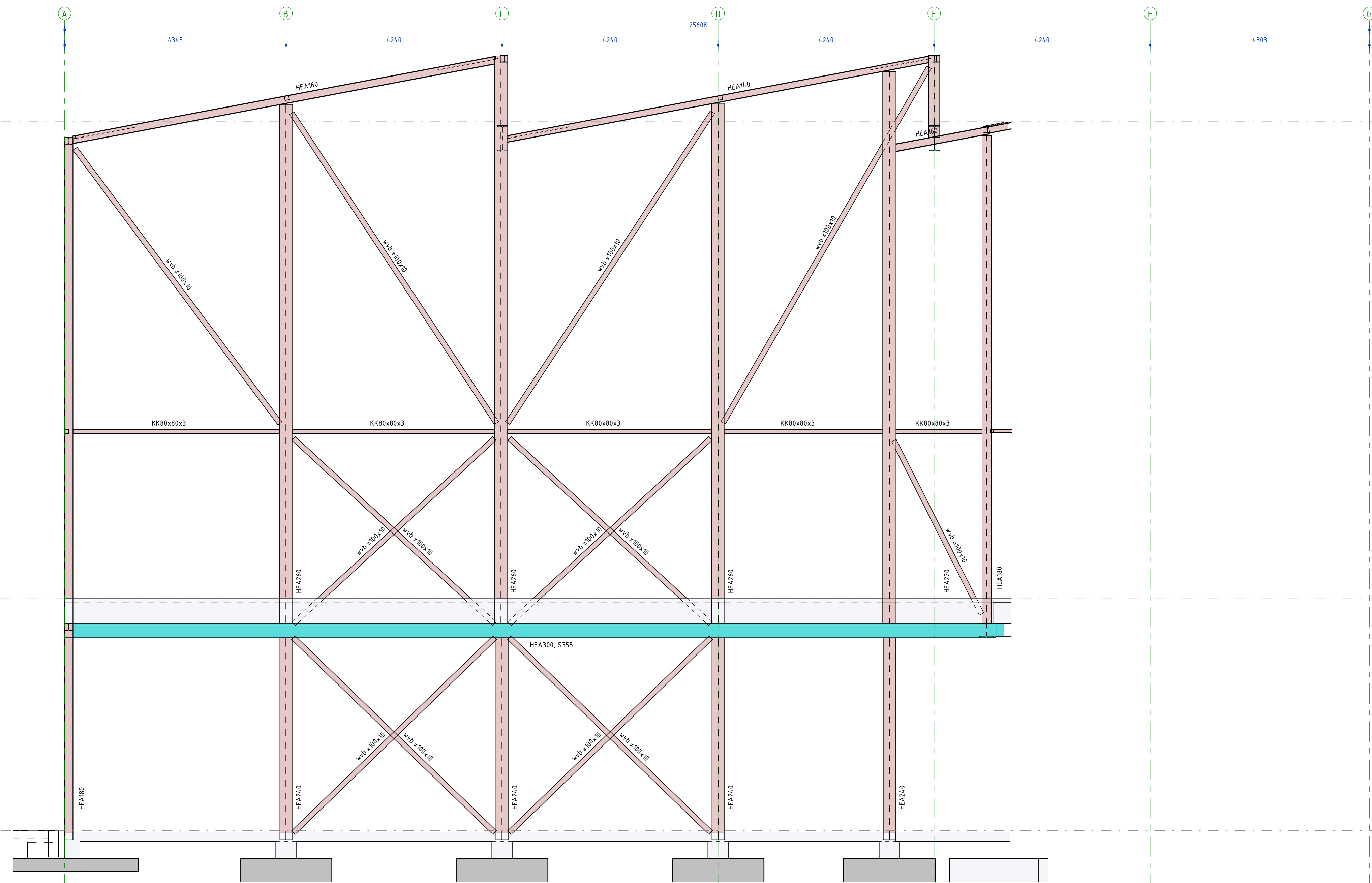
Aanzicht As 1
