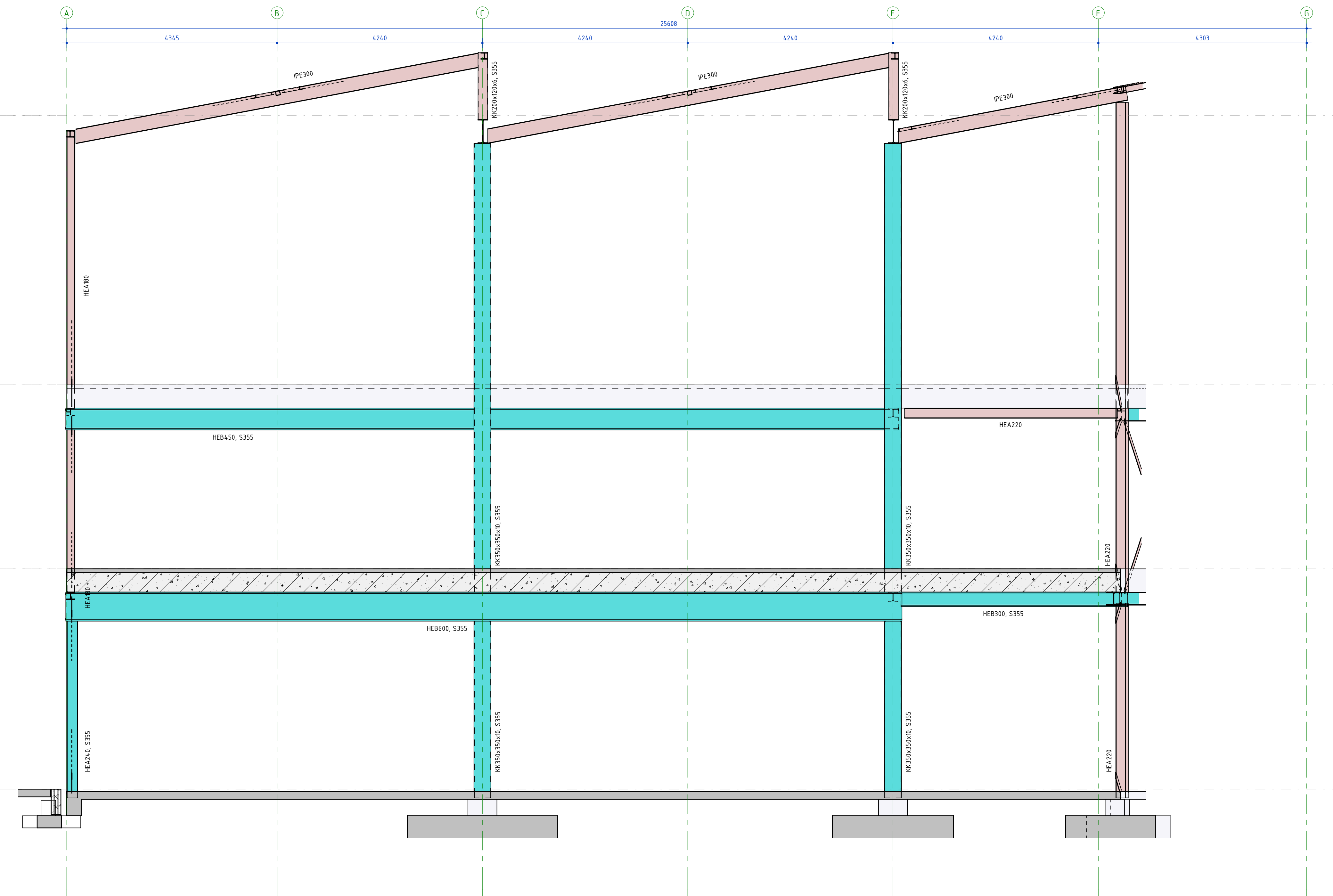
Aanzicht As 3
