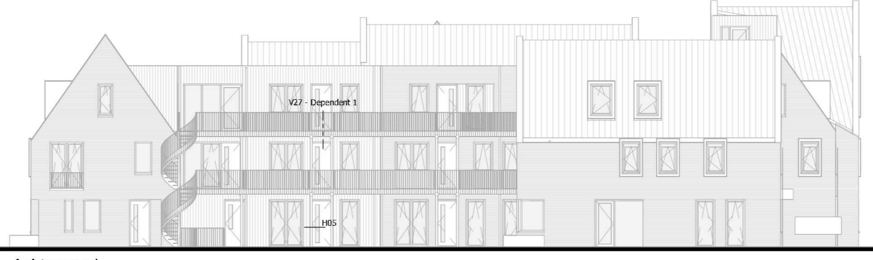
Achtergevel
