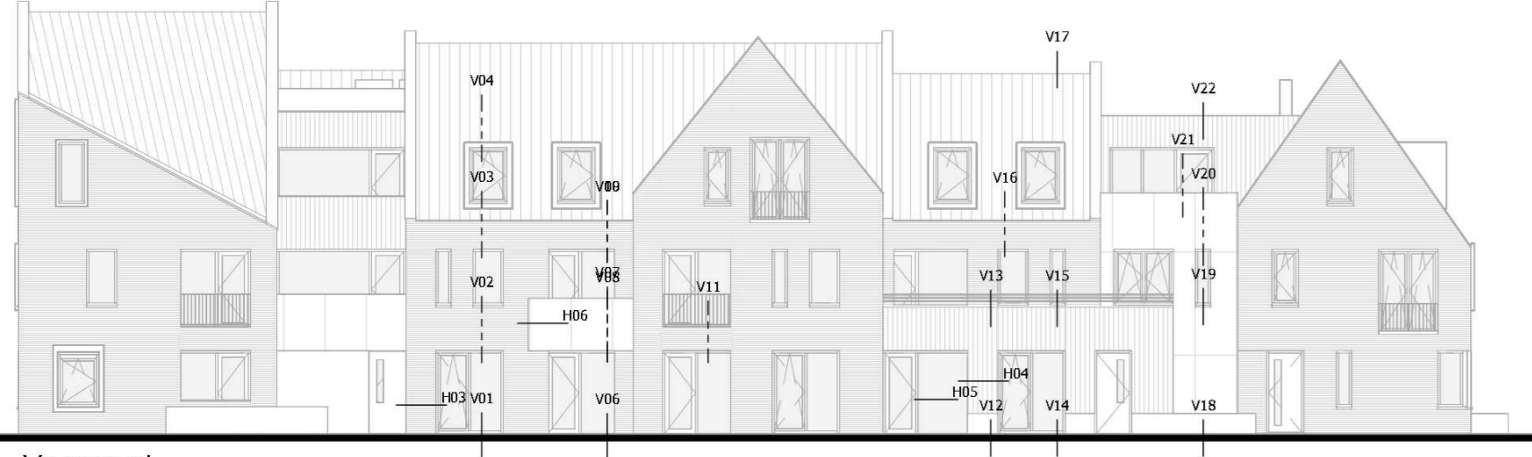
Voorgevel
