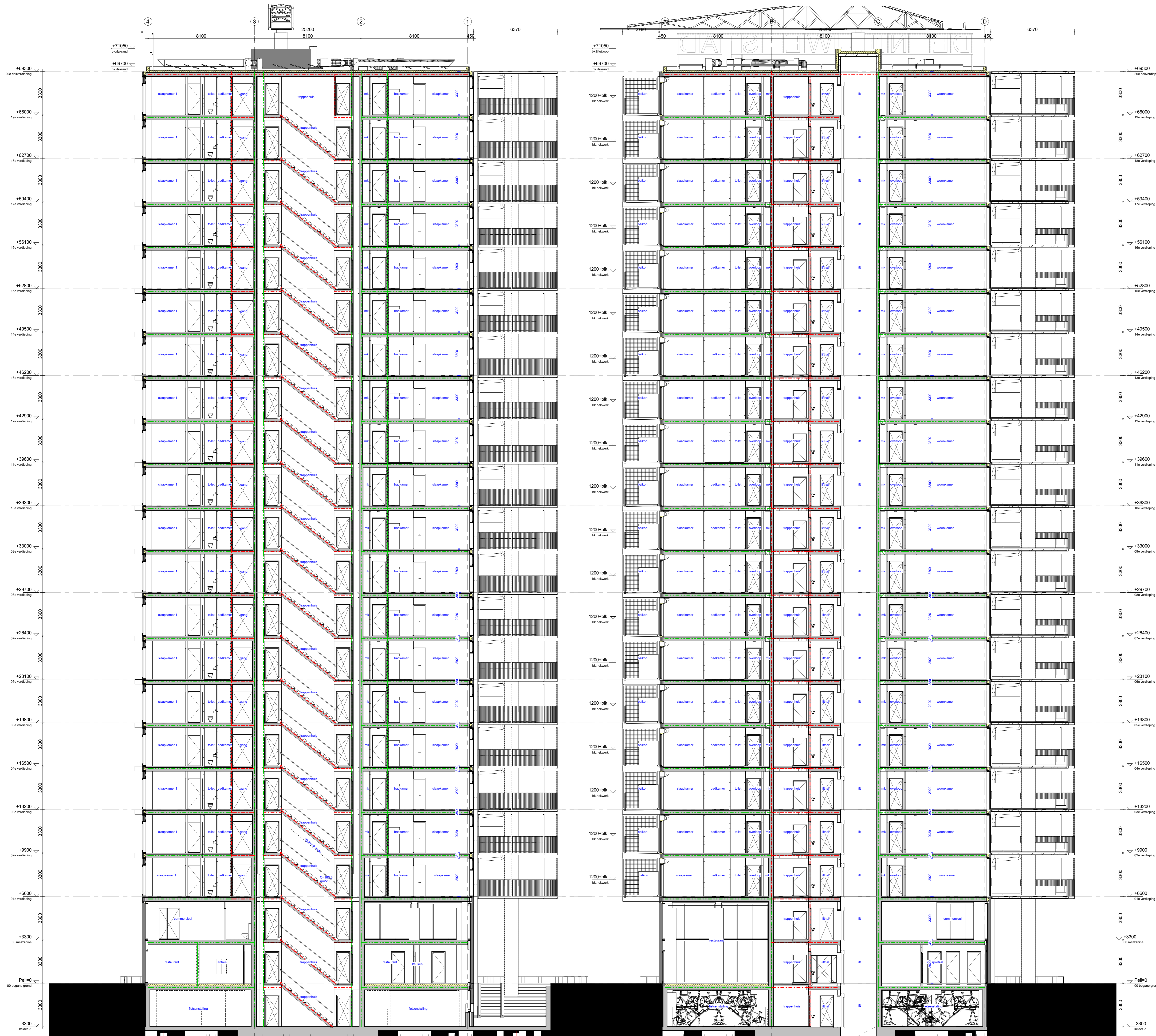
Doorsnede A-A'
