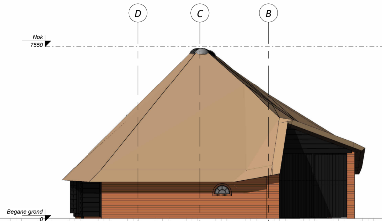
Achtergevel
