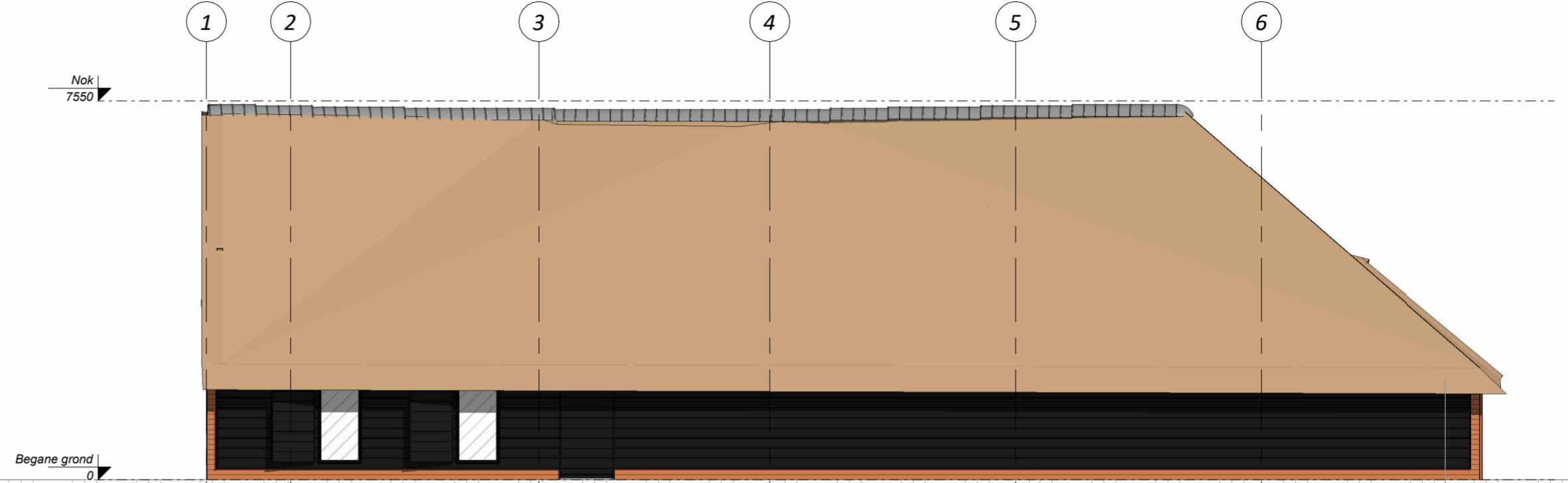
Rechter zijgevel
