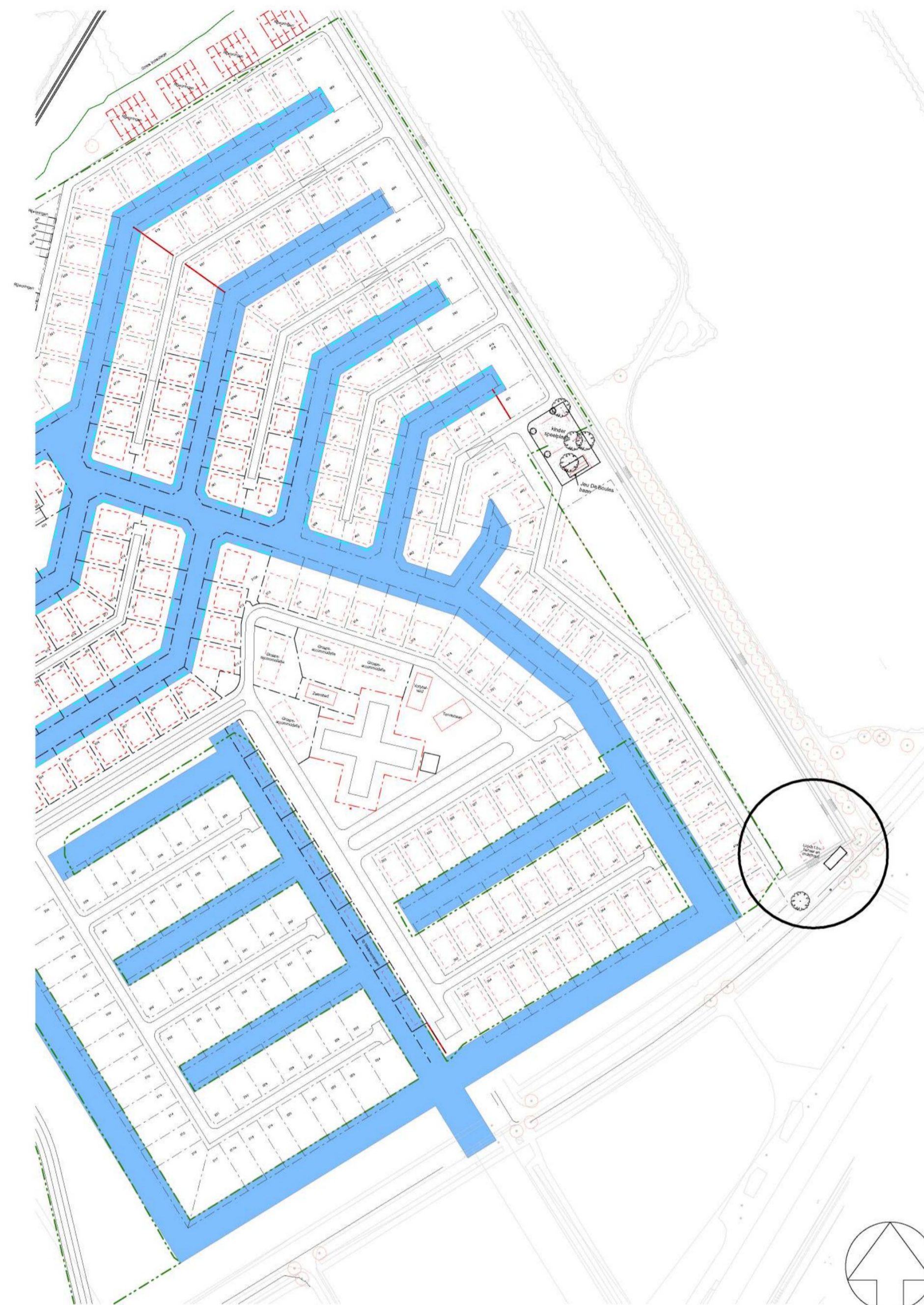
SITUATIE schaal 1:2500
