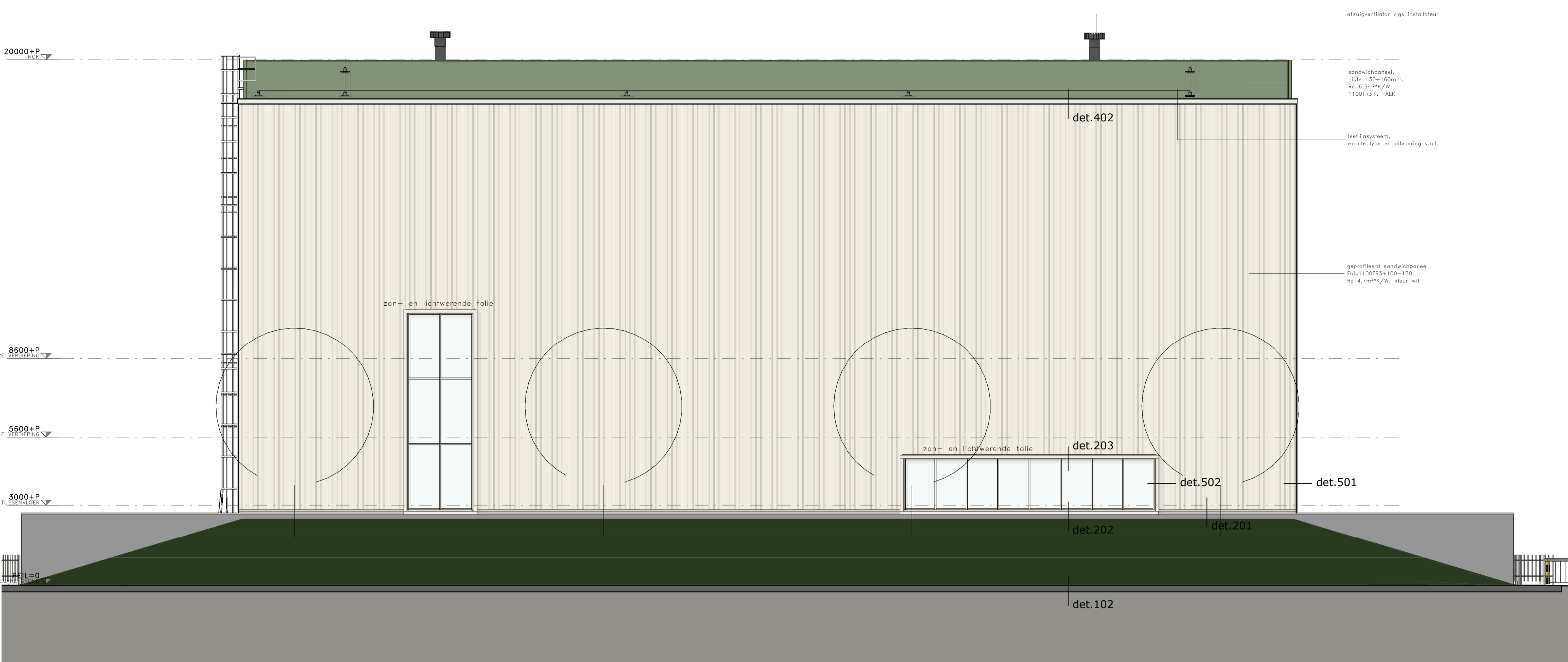
ZUID GEVEL
