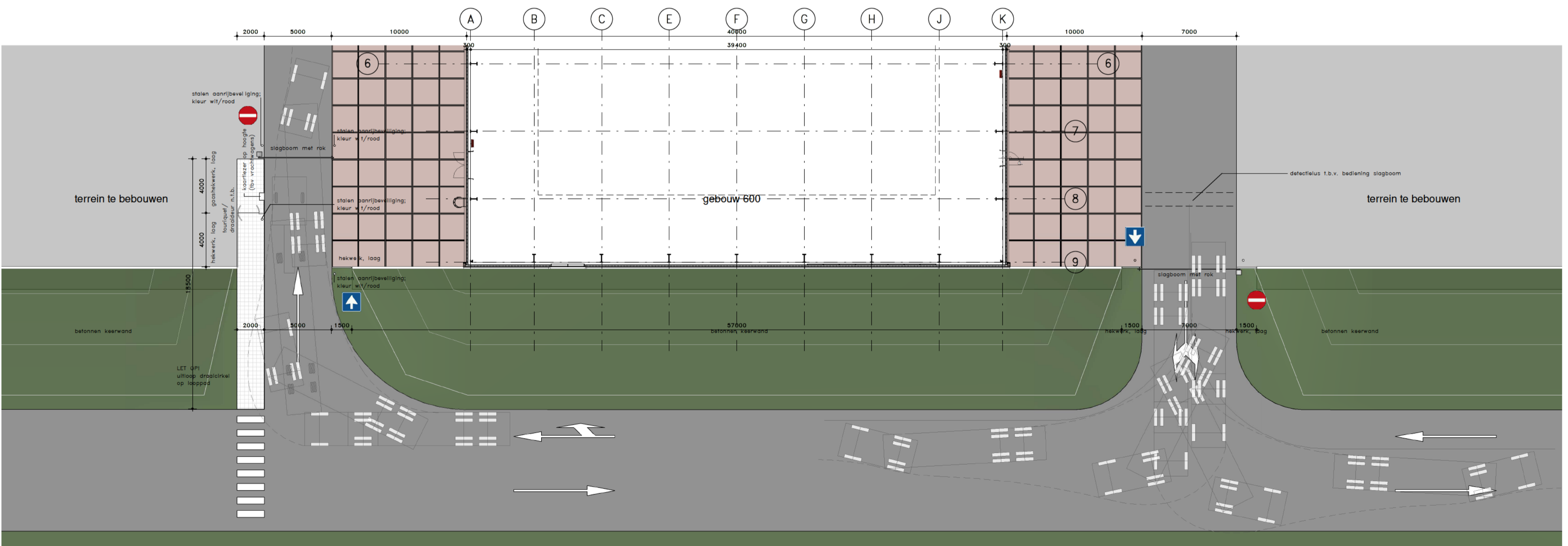
SITUATIE schaal 1:200
