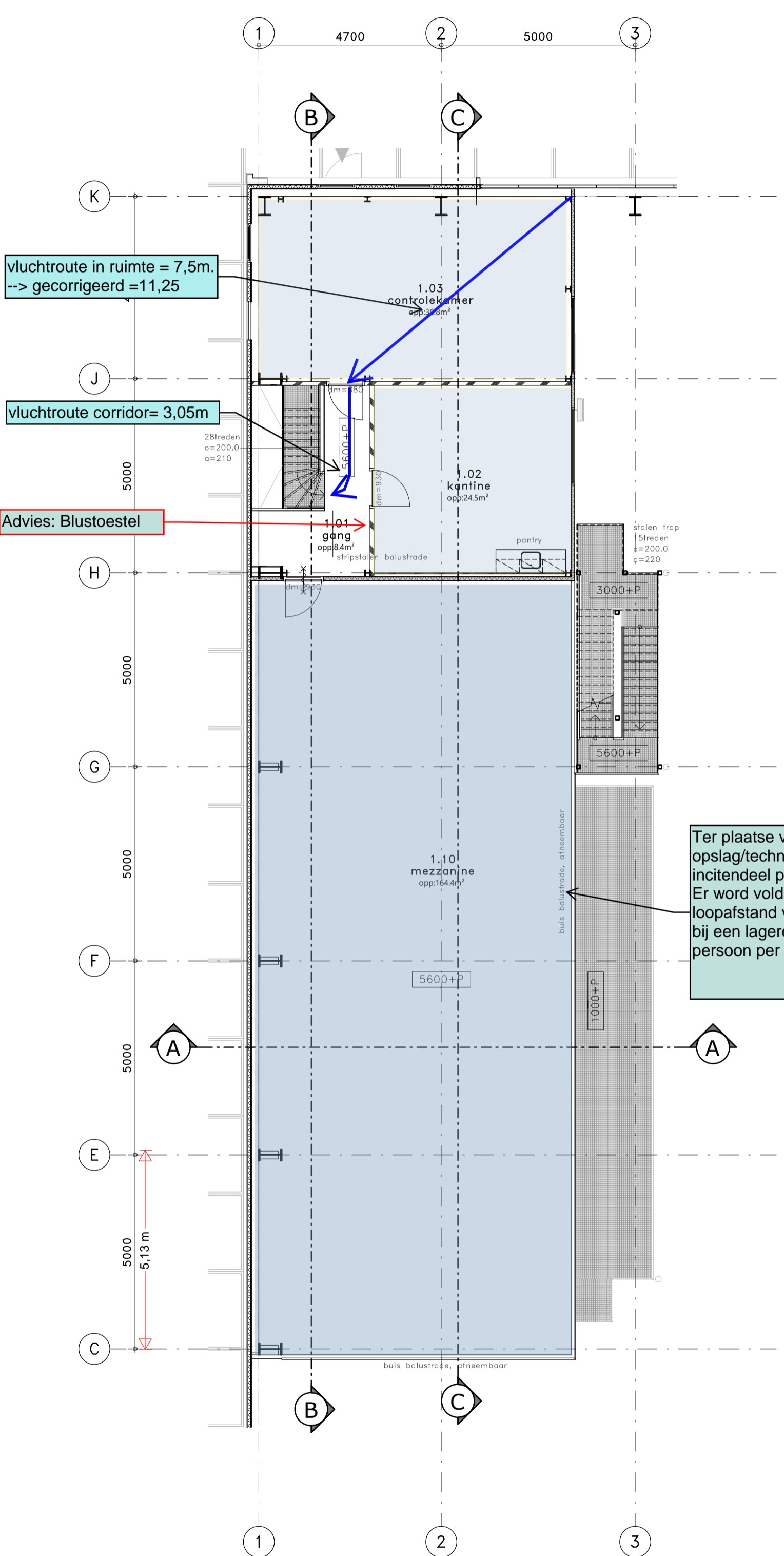
1e VERDIEPING
