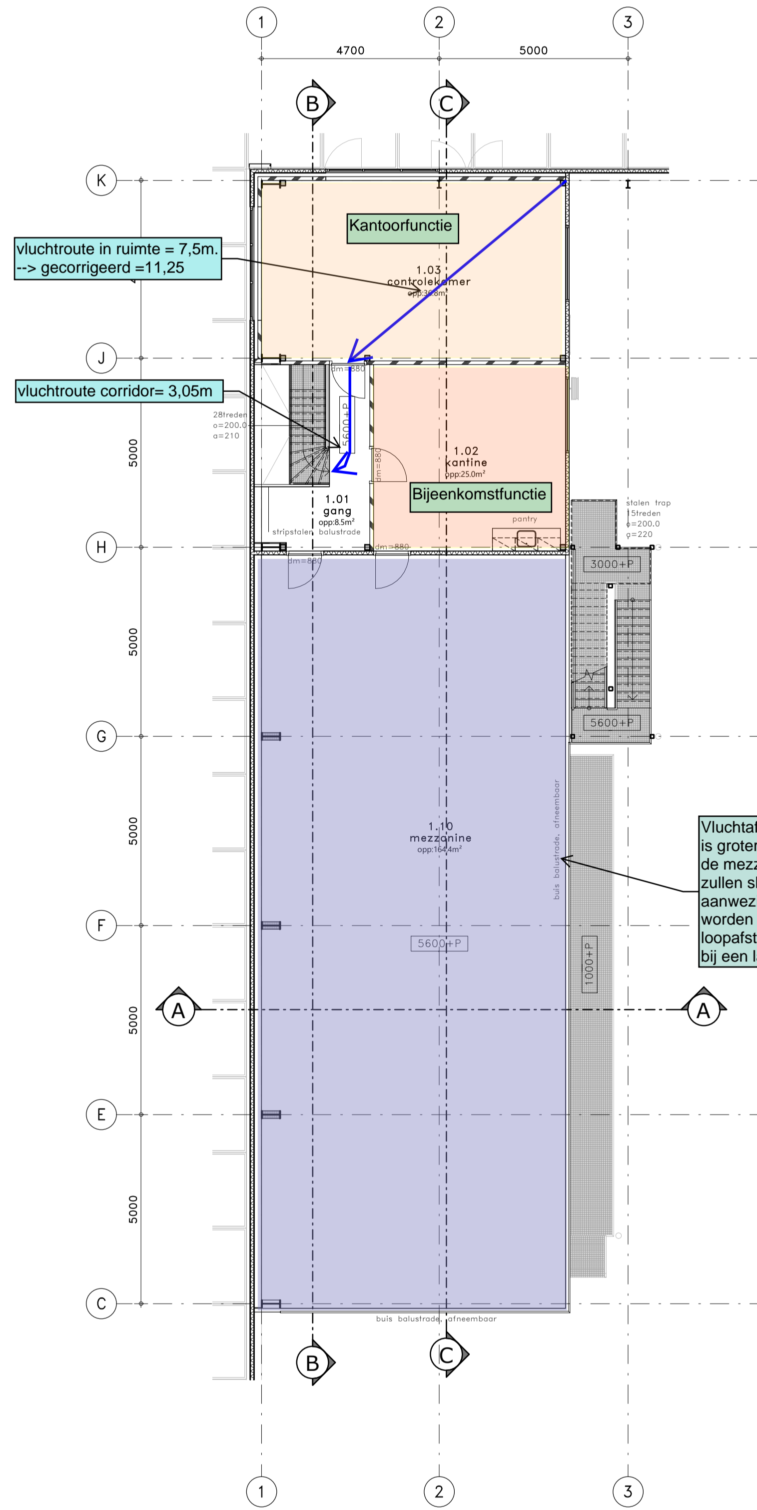
1e VERDIEPING
