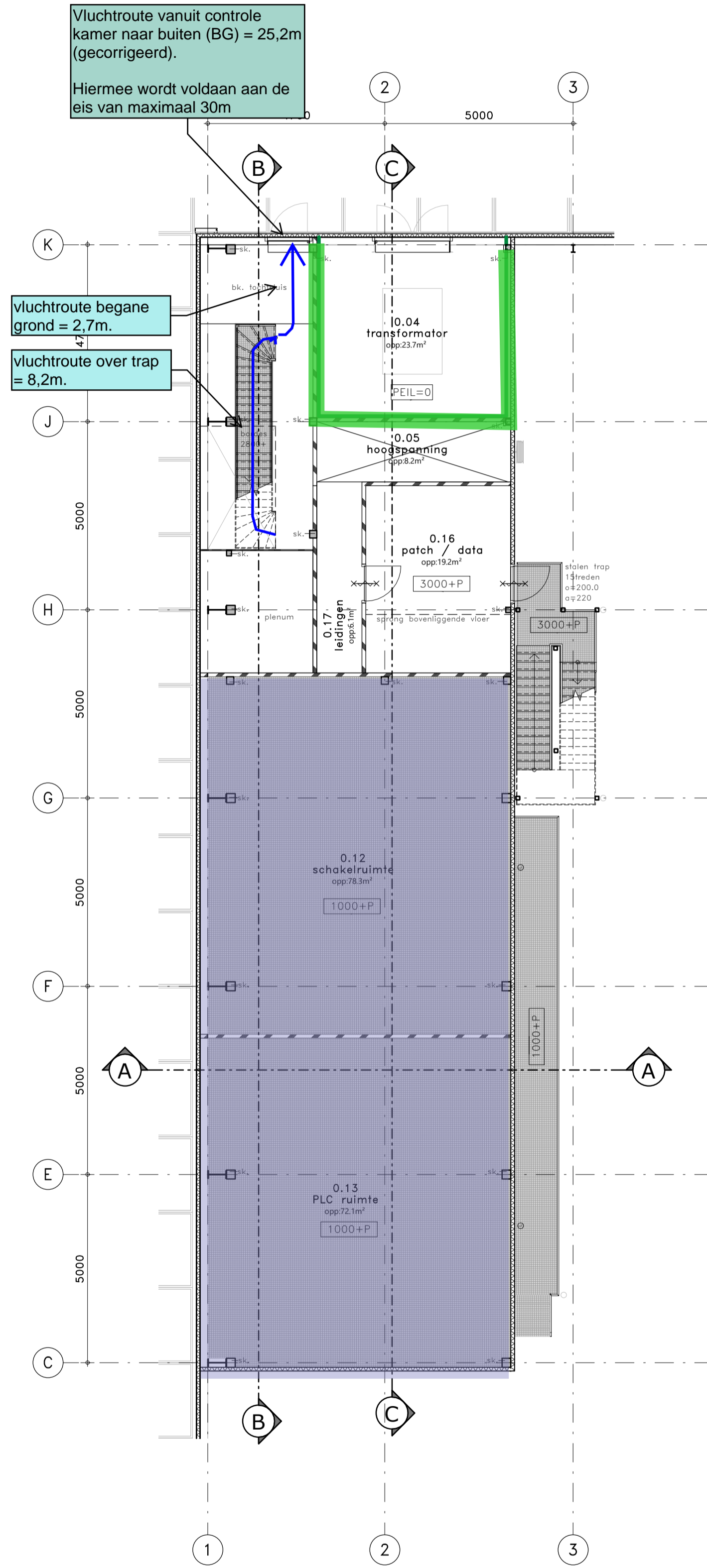
TUSSENVERDIEPING
