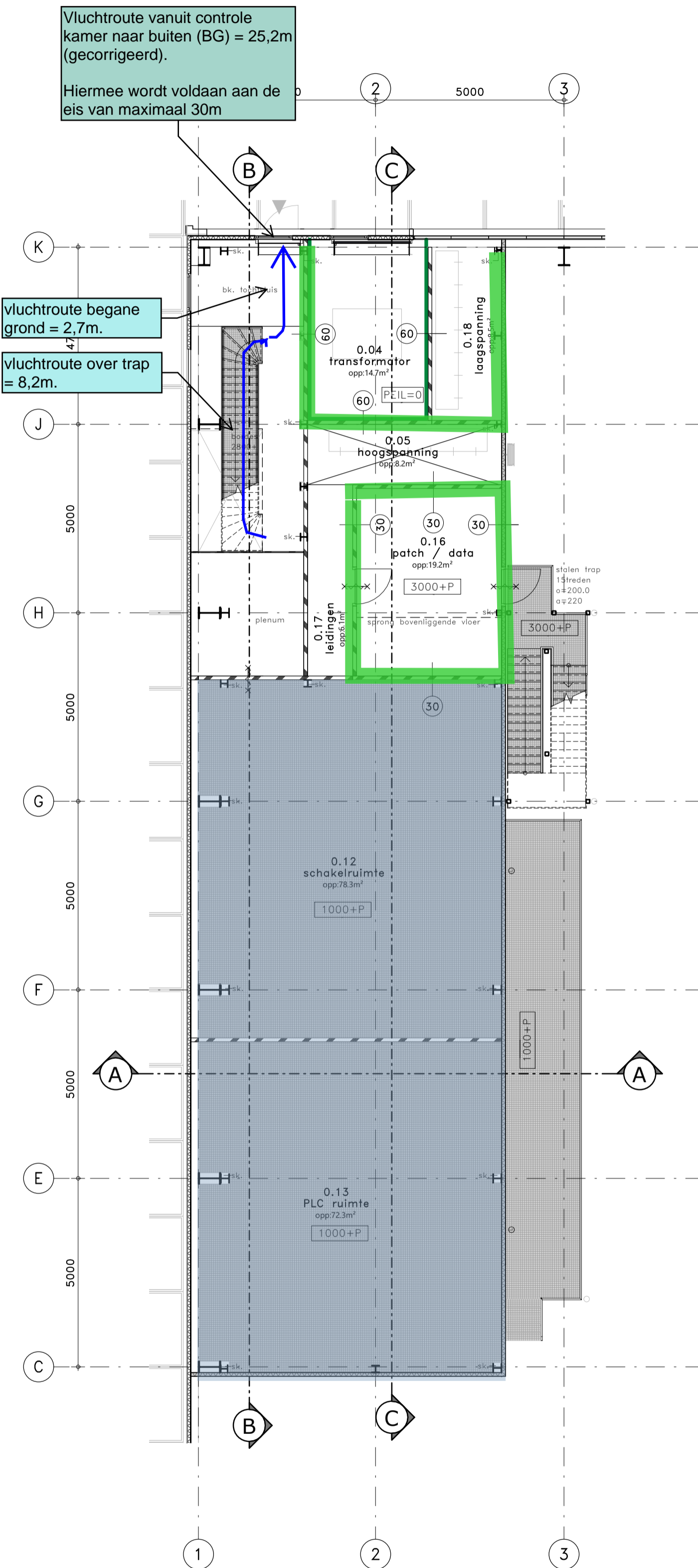
TUSSENVERDIEPING
