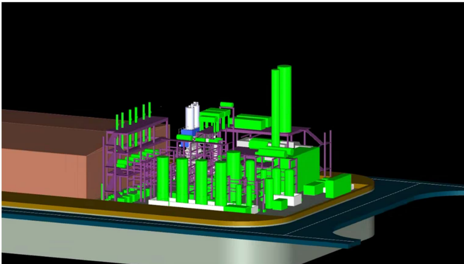
Figuur 4.1.2 3D-overzicht
