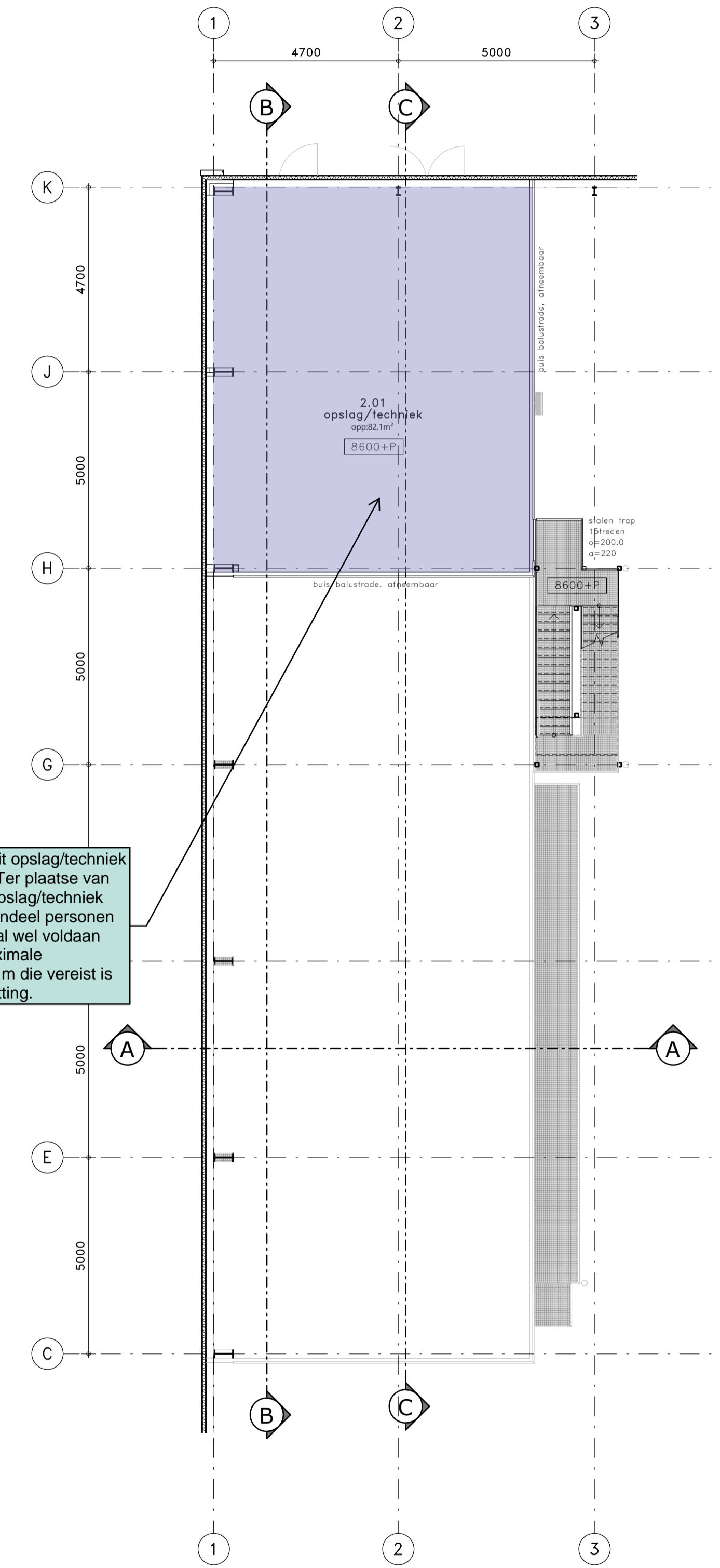
2e VERDIEPING
