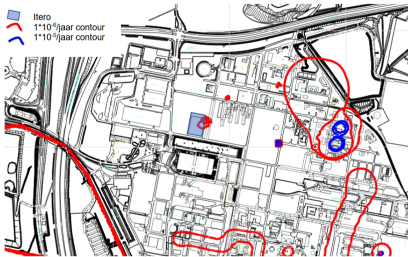
Figuur 2.2 Contour warmtestraling 35 kW/m 2
