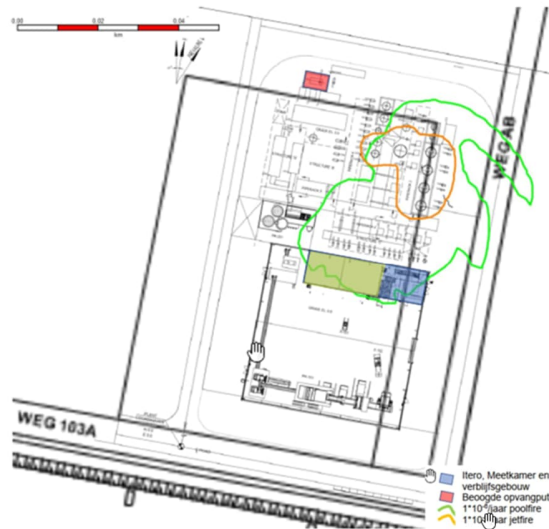
Figuur 2.3 Contour warmtestraling 35 kW/m 2 - uitverroot
