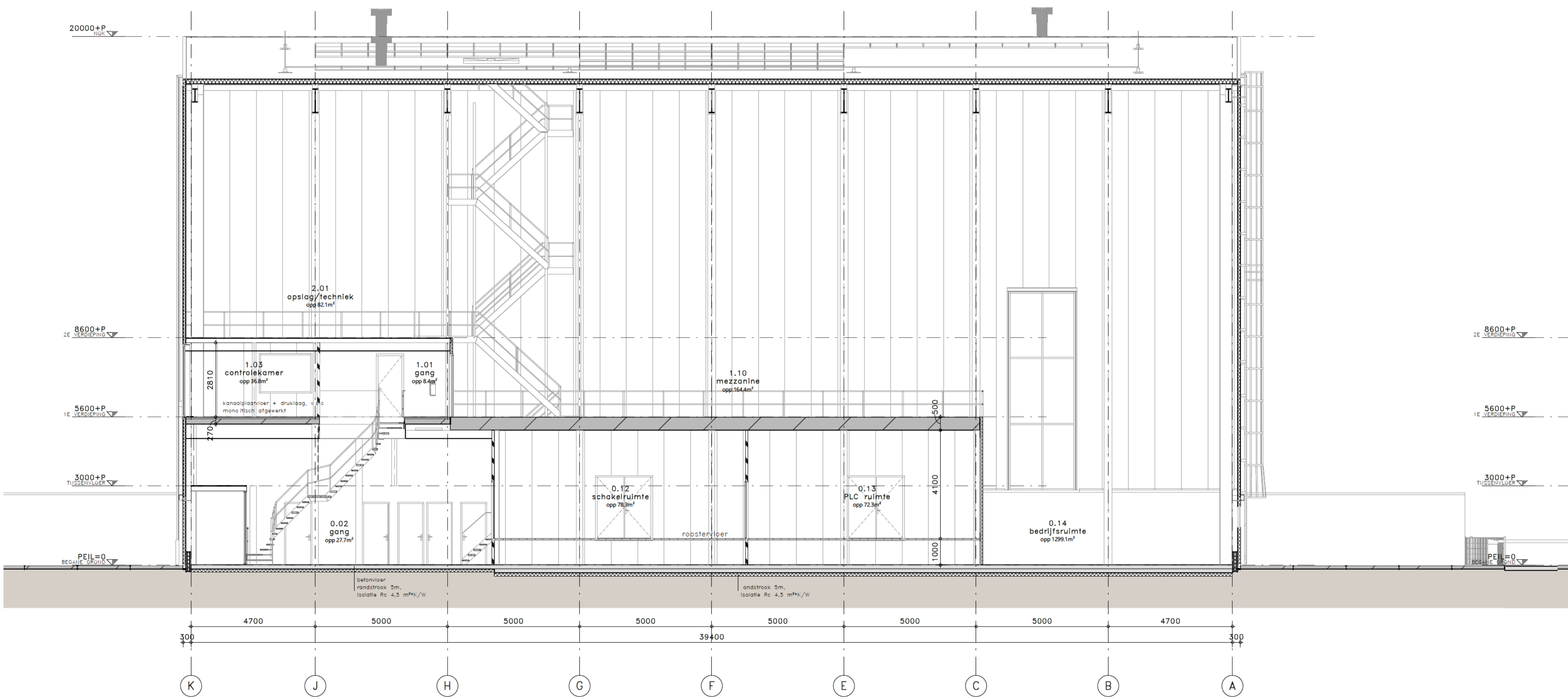
DOORSNEDE B-B
