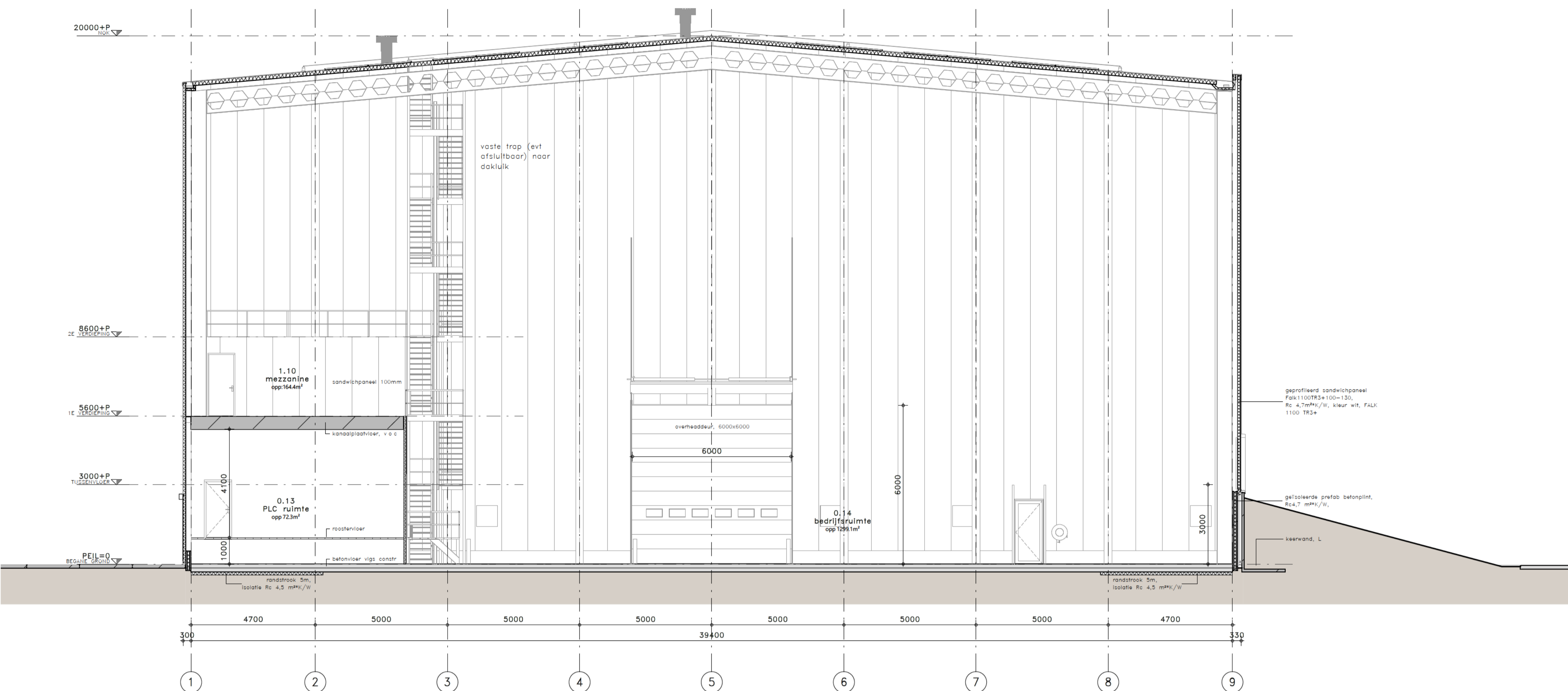
DOORSNEDE A-A
