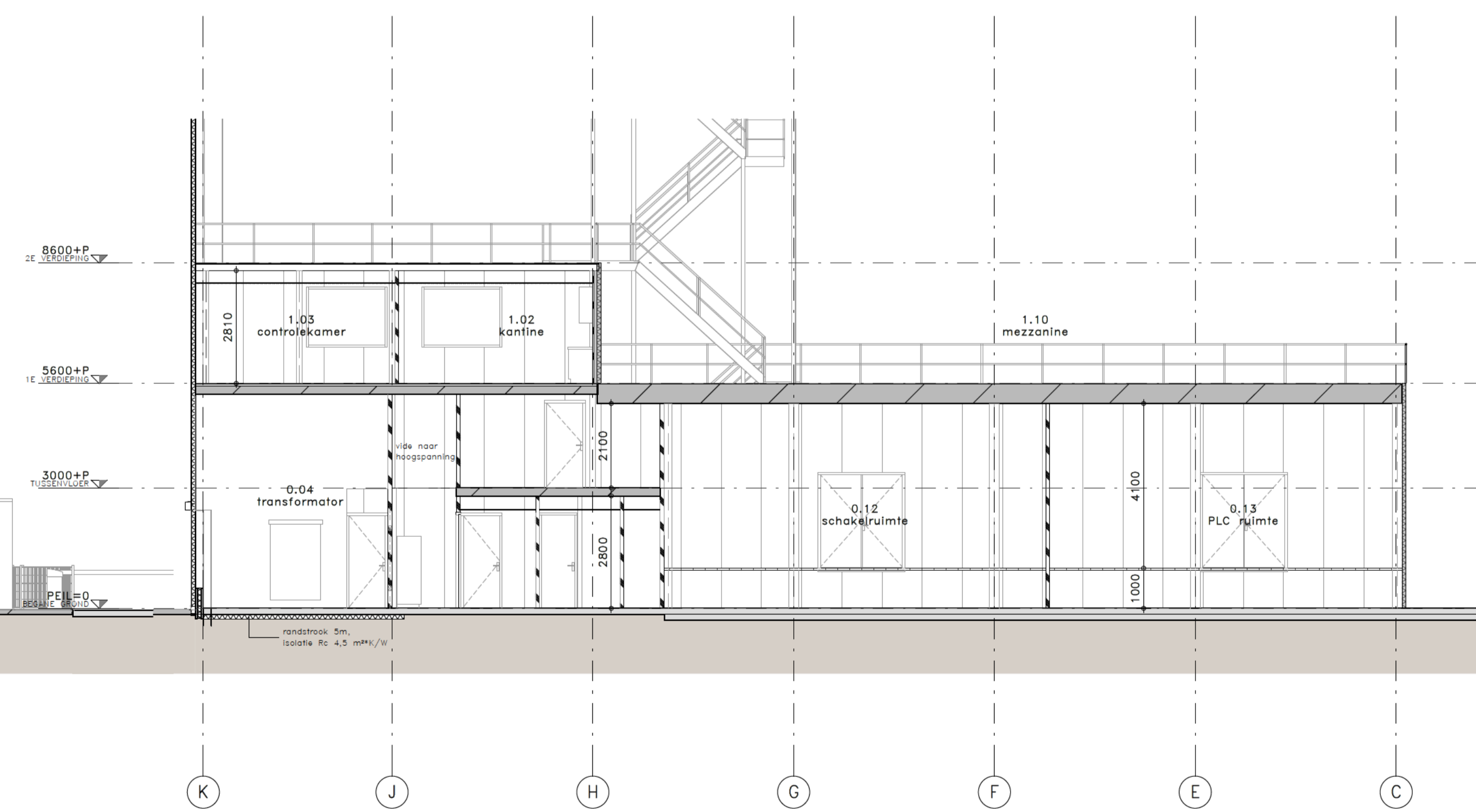
DOORSNEDE C-C
