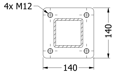
SECTION A-A Akkoord SCALE 1 : 5
