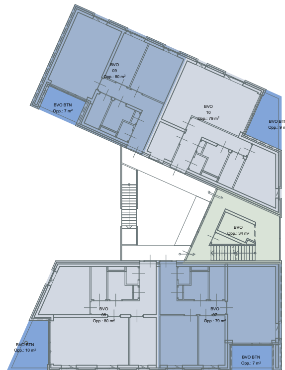
02 tweede verdieping
