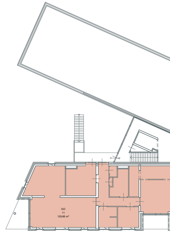
03 derde verdieping
