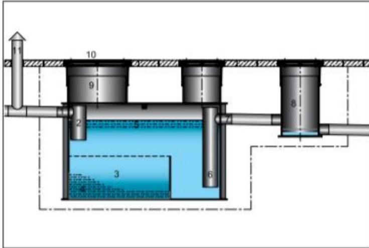
Afbeelding 1. Onderdelen van de vetafscheiderinstallatie
