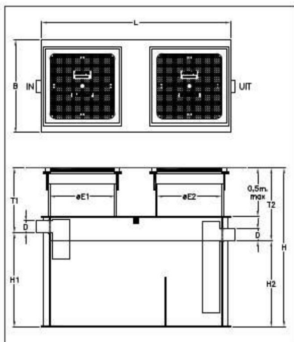
Afbeelding 2. Maattekening
